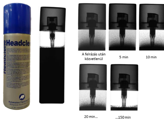
9. ábra. Egy felrázott tisztító sprayben kialakult hab ülepedése az idő függvényében
