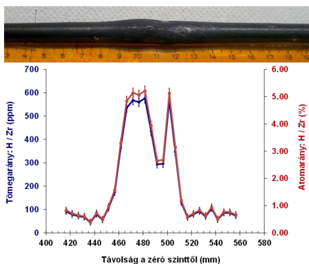
10. ábra. Egy, a CODEX-LOCA berendezéssel szimulált baleseti helyzet során megrongálódott E110G fűtőelem burkolat lokális hidrogéntartalma a hossz tengelye mentén, PGAI-NT módszerrel mérve.
