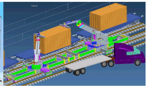
4. ábra: HCT modell Forrás: www.loxodon.com
