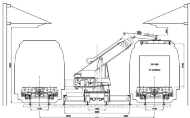
7. ábra: Az átrakási pont szelvénye azonos, vagy eltérő nyomtávú vasúti kocsik Forrás: Saját szerkesztés, 2019
