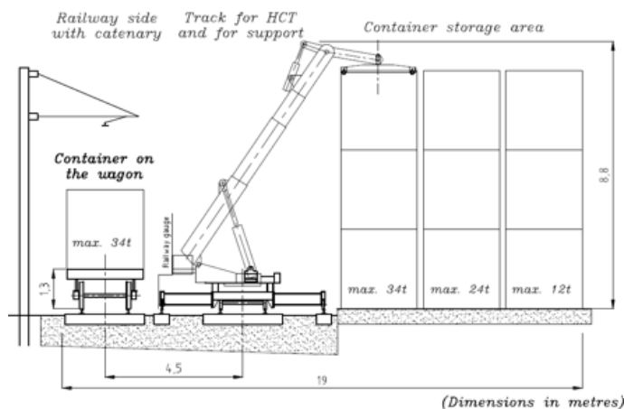
6. ábra: ITP szelvénye HCT-vel Forrás: Saját szerkesztés, 2019
