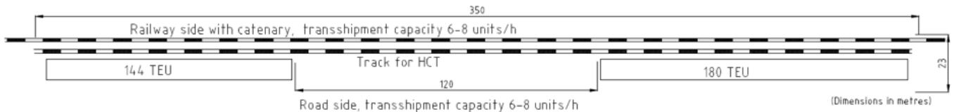
9. ábra: Kis kapacitású ITP HCT-vel
