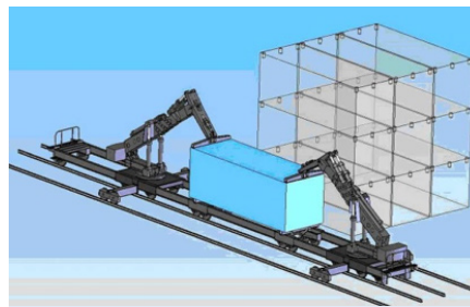
3. ábra: HCT modell Forrás: www.loxodon.com
