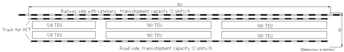
8. ábra: Közepes kapacitású ITP, 2 db HCT-vel
