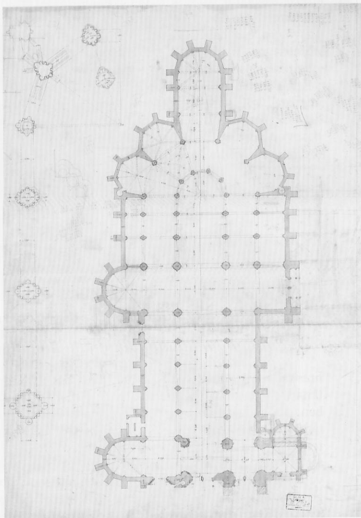
Henszlmann Imre – Henri-Eugène Leblan – Auguste Reimbeau: Lille, székesegyház, előtanulmányok (alaprajz), 1854. Forster Gyula Nemzeti Örökségvédelmi és Szolgáltató Központ, Tervtár
