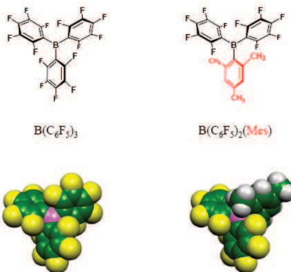
12. ábra: Meztíl-szubsztituált borán: a savas centrum fokozottan árnyékolt
