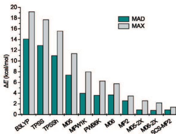
6. ábra: Különböző módszerek átlagos (MAD) és maximális (MAX) hibái
