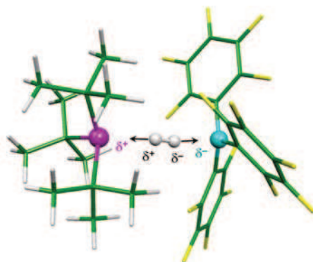
7. ábra: Heterolitikus H 2 hasítás a frusztrált PR 3 /BAr 3 pár segítségével
