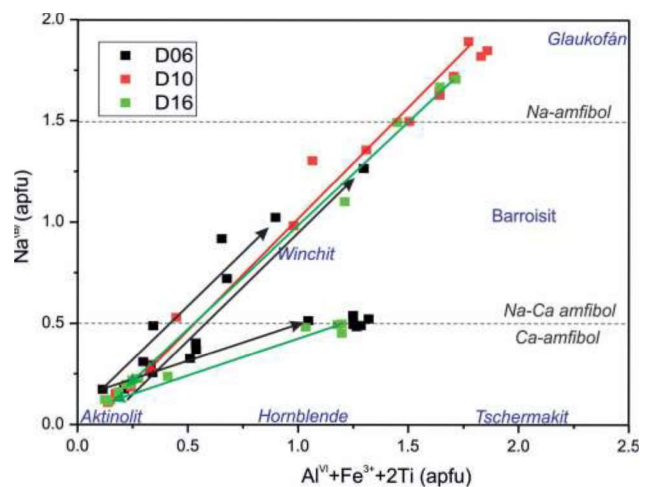
5. ábra – Amphibolok kémiai összetétele a kékpala kőeszközökben az Al^{VI}+Fe^{3+}+2Ti vs Na^{(B)} (apfu: atoms per formula unit) diagramon ábrázolva, nyílal jelezve a mag és szegély közötti fázisváltozásokat
