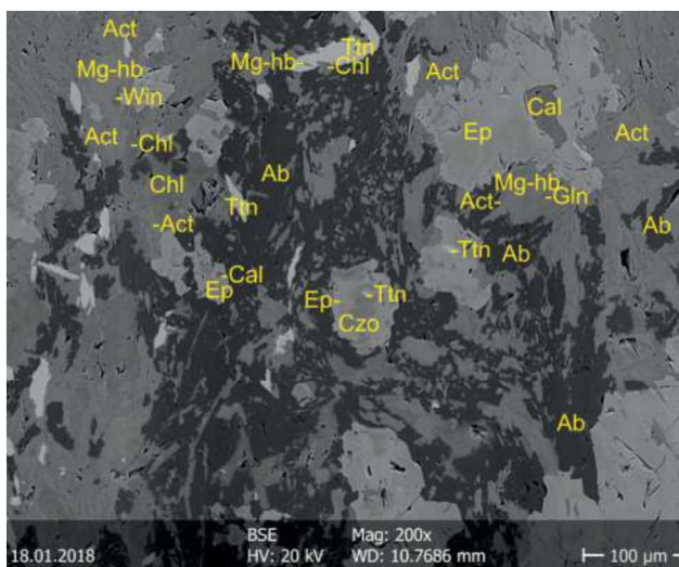
3. ábra – A D16 kőbaltá BSE képe Ásványnév rövidítések: Gln: glaukofán; Win: winchit; F-win: ferriwinchit; Mg-hb; magneziohornblende; Act: aktinolit; Ab: albit; Ep: epidot; Czo: klinozoisit; Ttn: titanit; Chl: klorit; Qtz: kvarc; Ph: fengit; Cal: kalcit
