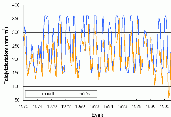
3. ábra: Az 1972-1992 időszakra vonatkozó mért és szimulált \Theta -k évi menete a Debreceni Observatórium területén. Az alkalmazott modell: vízháztartás szimulálása: csöbör modell; a PET parametrizálása: THORNTHWAITE (1948); a \beta parametrizálása: exponenciális összefüggés (MINTZ és WALKER, 1993); numerikus séma: módosított másodrendű implicit séma.
