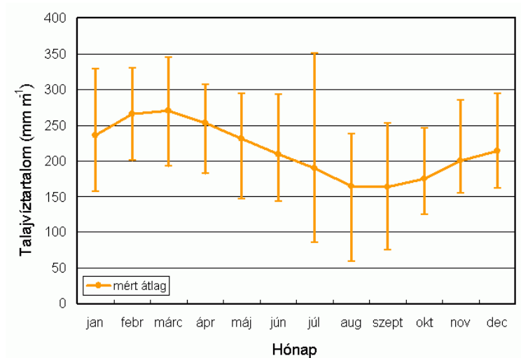
4b. ábra: A Debreceni Observatórium által mért talajvíztartalom átlagos évi menete és szórása vályog textúrájú talaj esetén.
