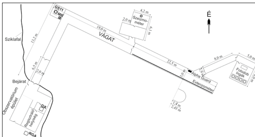
2. ábra. Az observatórium alaprajza a vágat méreteivel, a régi és jelenlegi műszerek elhelyezésével
