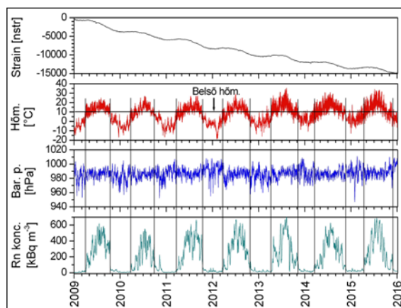
19. ábra. Extenzométer, külső hőmérséklet, mikrobarográf- és radonkoncentráció-mérési eredmények az observatóriumban 2009 és 2016 között.
