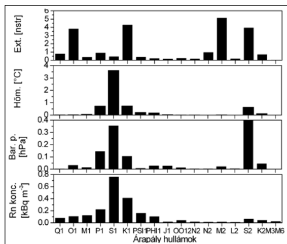
20. ábra. Extenzométer, külső hőmérséklet, mikrobarográf és radonkoncentráció árapály-kiértékelésének eredményei az observatóriumban 2009 és 2016 között.
