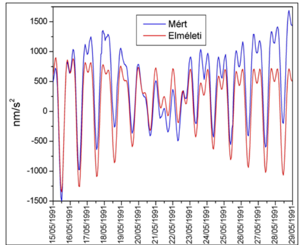
11. ábra. Az átalakított GS-11 graviméter által regisztrált és az adott időszakra számított elméleti árapálygörbe
