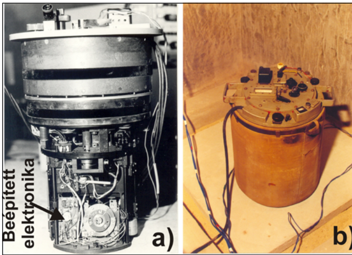
10. ábra. a) A GS-11 átalakított graviméter belseje b) A graviméter a regisztrálás helyén
