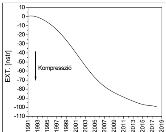
17. ábra. Az SGO-ban regisztrált tektonikai deformáció 1991 és 2018 között
