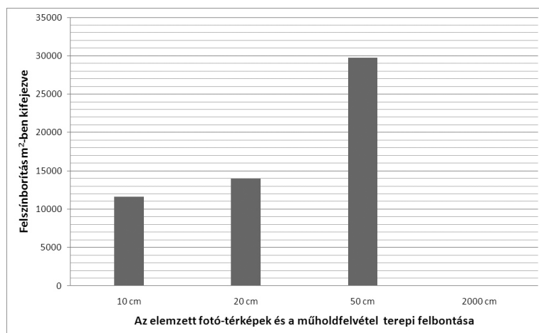
4. ábra A tájsebek, humuszos réteget veszített talajfelszínek (kopárok) által fedett területek lehatárolásának eredménye különböző terepi felbontású felvételekből kiindulva Figure 4. Area of identified degraded (damaged) landscapes and bare soils (lost topsoil) on aerial photographs at different field resolution
