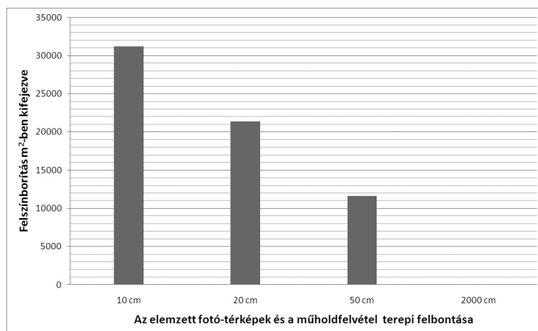
3. ábra A földutak és tömörödött kopárok által fedett területek lehatárolásának eredménye különböző terepi felbontású felvételekből kiindulva Figure 3. Area of identified dirt roads and solid bare soils on aerial photographs at different field resolution
