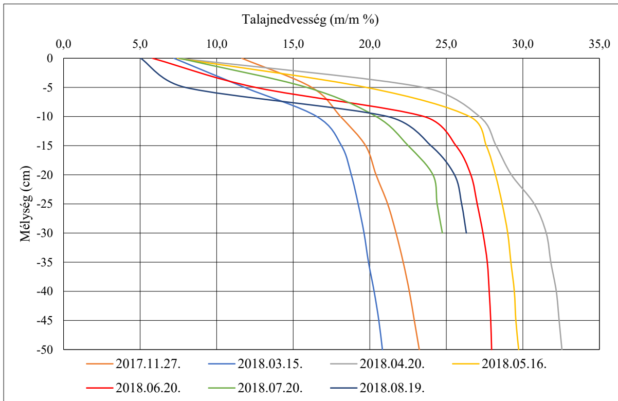
M3. 50. ábra: A talajnedvesség adatok időbeli eloszlása, a sekély kultivátoros kezelésben (Józsefmajor, 2018)
