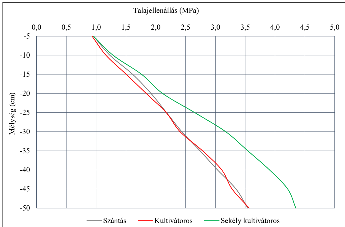
8. ábra: Az átlagos talajellenállás (MPa) különböző művelési kezelésekből (Lukács, 2017)
