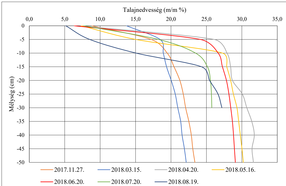
M3. 51. ábra: A talajnedvesség adatok időbeli eloszlása, a direktvetés kezelésben (Józsefmajor, 2018)
