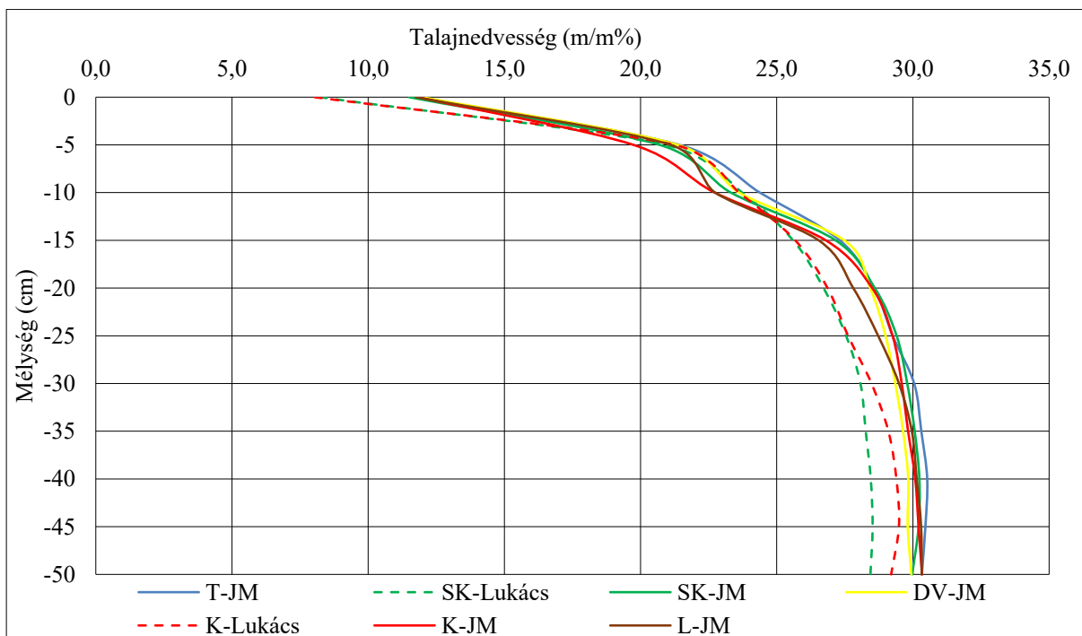
M3. 69. ábra: Talajnedvesség (m/m%) alakulása eltérően művelt talajokban, két termőhelyen, (2017)
