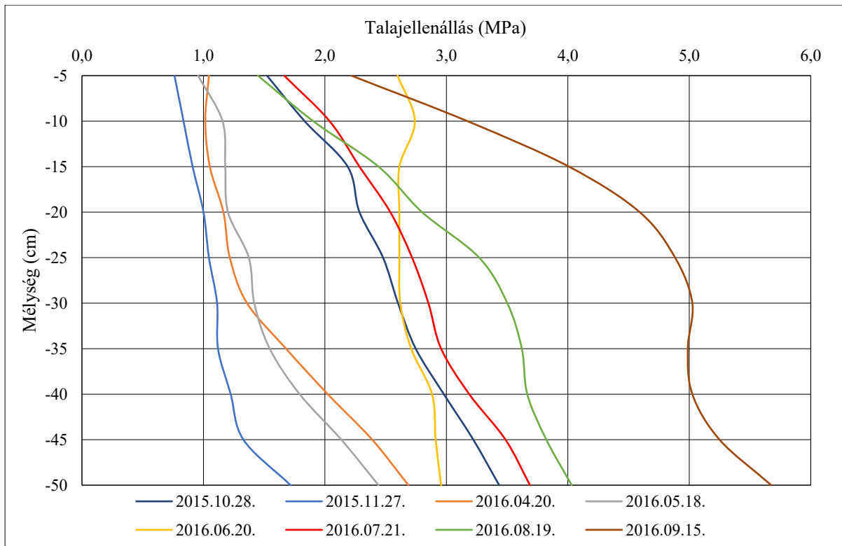
M3. 15. ábra: A talajellenállás adatok időbeli eloszlása, a lazításos kezelésben (Józsefmajor, 2016)
