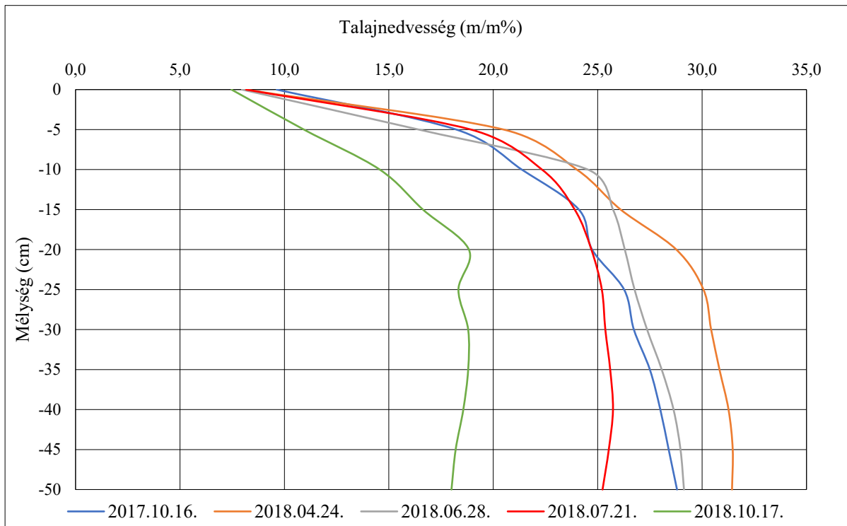
M3. 34. ábra: A talajnedvesség adatok időbeli eloszlása, a kultivátoros kezelésben (Lukács, 2018)
