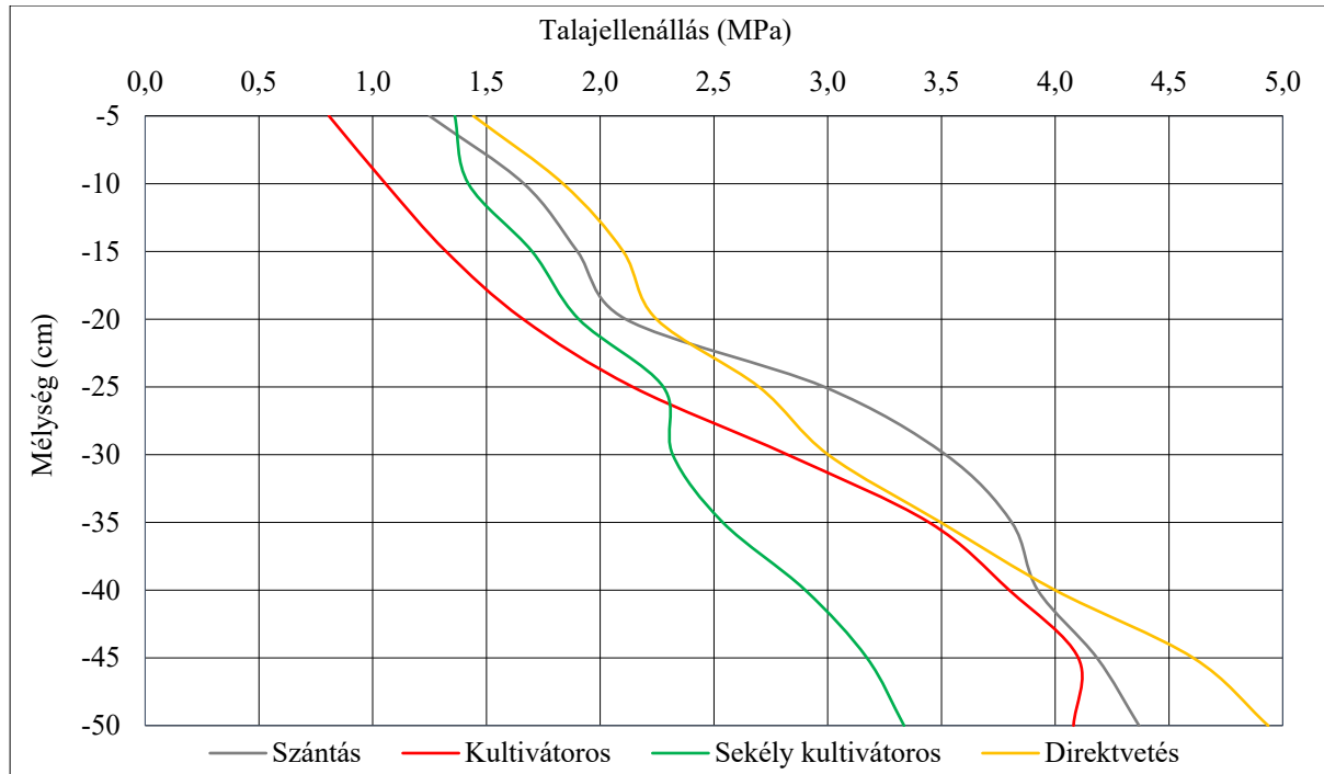
9. ábra: Az átlagos talajellenállás (MPa) különböző művelési kezeléseknél (Lukács, 2018)
