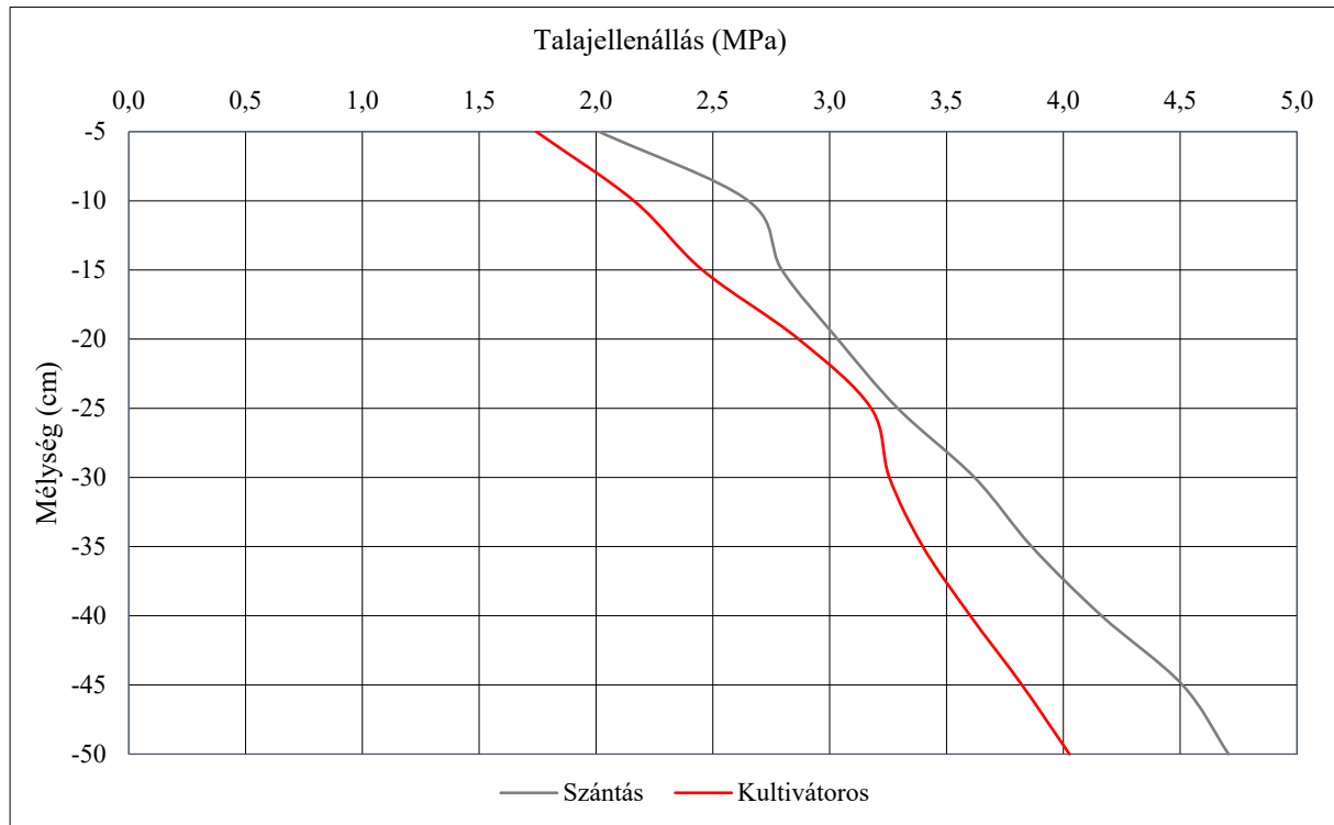
7. ábra: Az átlagos talajellenállás (MPa) különböző művelési kezeléseknél (Lukács, 2016)
