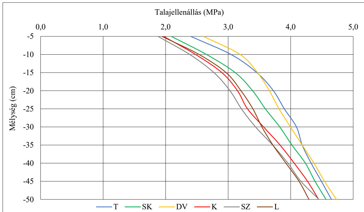
11. ábra: Az átlagos talajellenállás (MPa) különböző művelési kezeléseknél (Józsefmajor, 2017) Megjegyzés: a méréskor az átlag talajnedvesség a tárcsás 25,8 m/m%, a sekély kultivátoros 25,4 m/m%, a direktvetés 25,2 m/m%, a kultivátoros 25,0 m/m%, a szántásban 25,3 m/m% és a lazításos kezelésben 25,1 m/m%. Kezelések: T: tárcsás, SK: sekély kultivátoros, DV: direktvetés, K: kultivátoros, SZ: szántás, L: lazításos
