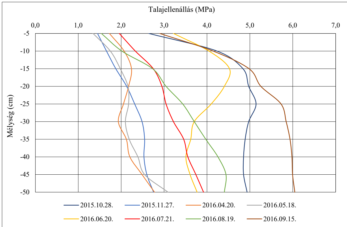
M3. 10. ábra: A talajellenállás adatok időbeli eloszlása, a tárcsás kezelésben (Józsefmajor, 2016)
