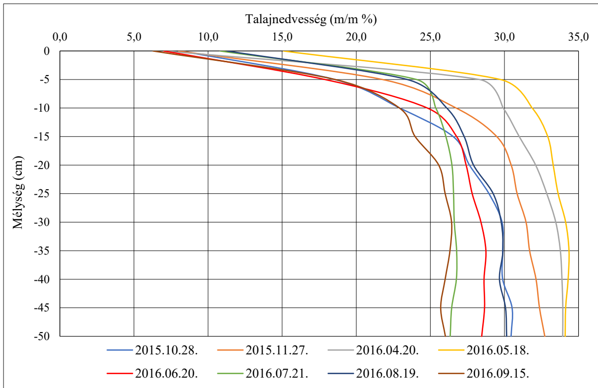
M3. 38. ábra: A talajnedvesség adatok időbeli eloszlása, a sekély kultivátoros kezelésben (Józsefmajor, 2016)
