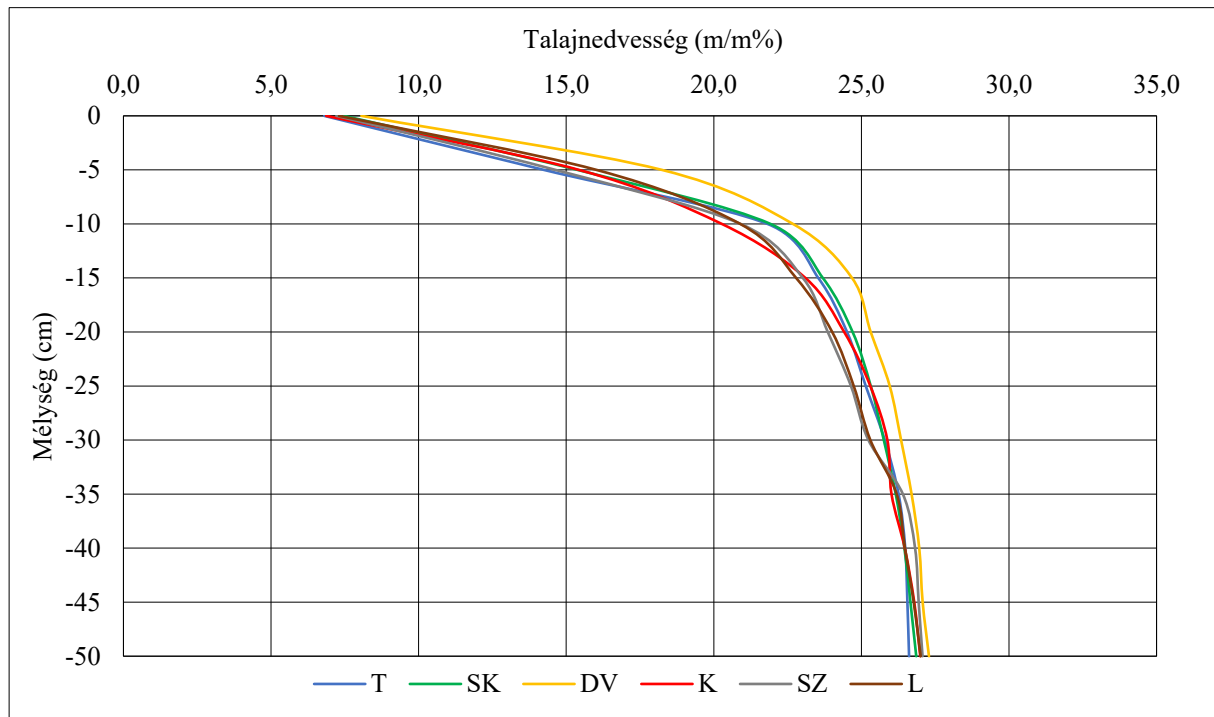
18. ábra: Az átlagos talajnedvesség (m/m%) különböző művelési kezeléseken (Józsefmajor, 2018) Kezelések: T: tárcsás, SK: sekély kultivátoros, DV: direktvetés, K: kultivátoros, SZ: szántás, L: lazításos
