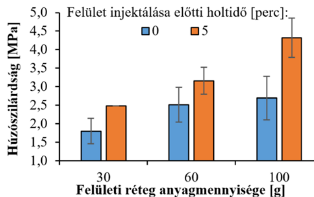
10. ábra: Húzószilárdság a felületi réteg vastagsága és a rétegek öntése között eltelt holtidő függvényében
