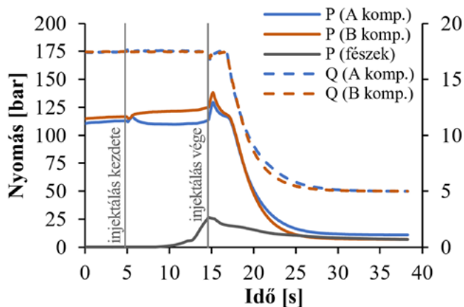
3. ábra: DU1 injektálási ciklus – előgyártmány készítése (P: nyomás, Q: tömegáram)
