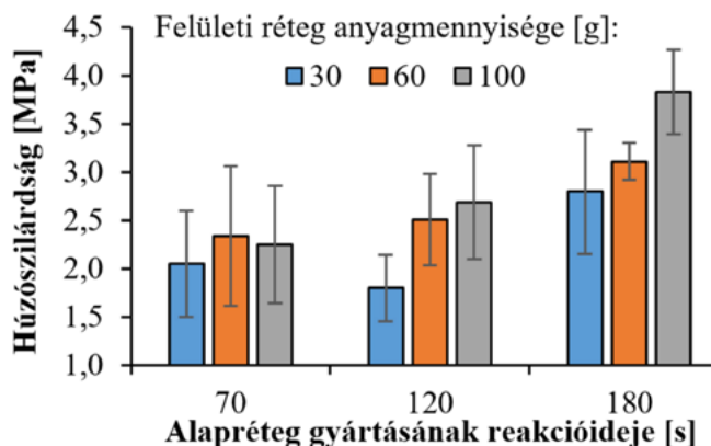
9. ábra: Húzószilárdság a felületi réteg vastagsága és az alaprég reakcióideje függvényében
