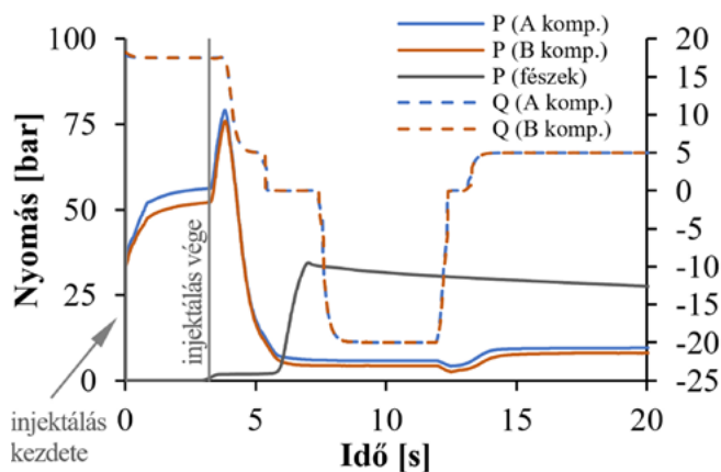
4. ábra: DU2 injektálási ciklus – felületi réteg készítése (P: nyomás, Q: tömegáram)
