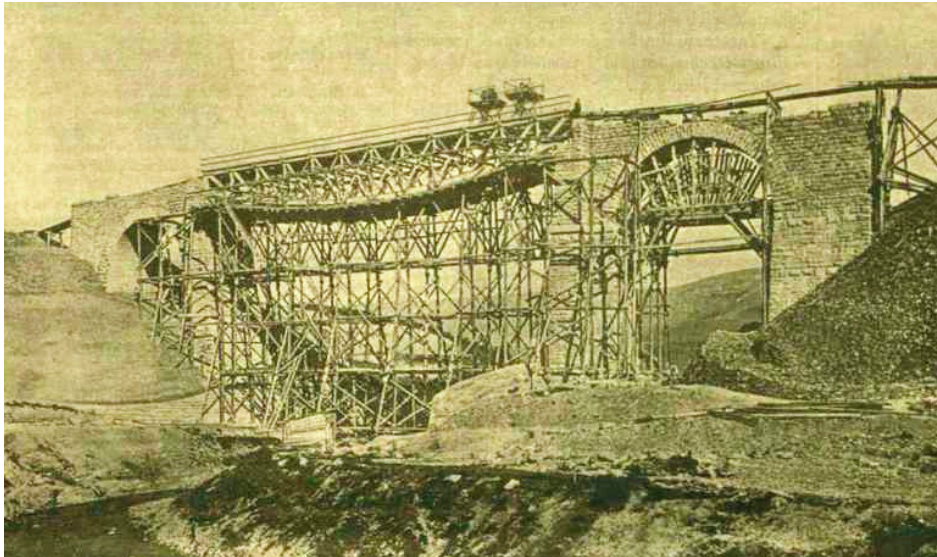
29. kép A munkács–beszki viadukt (Dörre Tivadar rajza, 1884–1887)
