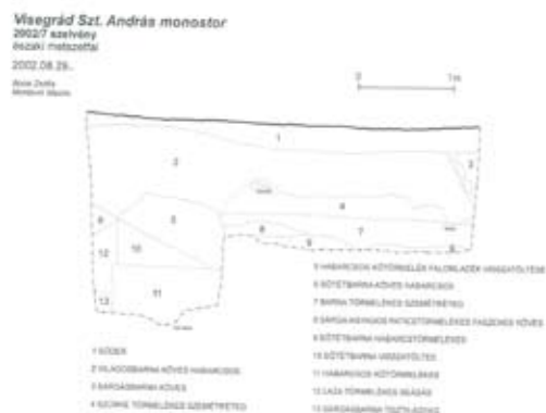
11. A 2002/7. szelvény északi metszetzala a gótikus szentély kiszedett alapozásának árkáival
