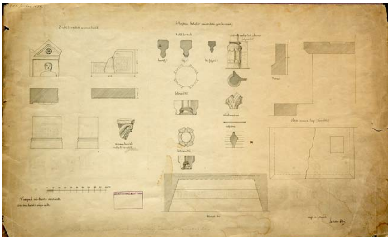
3. Szezhlo Ottó felmérési rajzai a Szt. András monostorból előkerült kőfaragványokról (1894)
