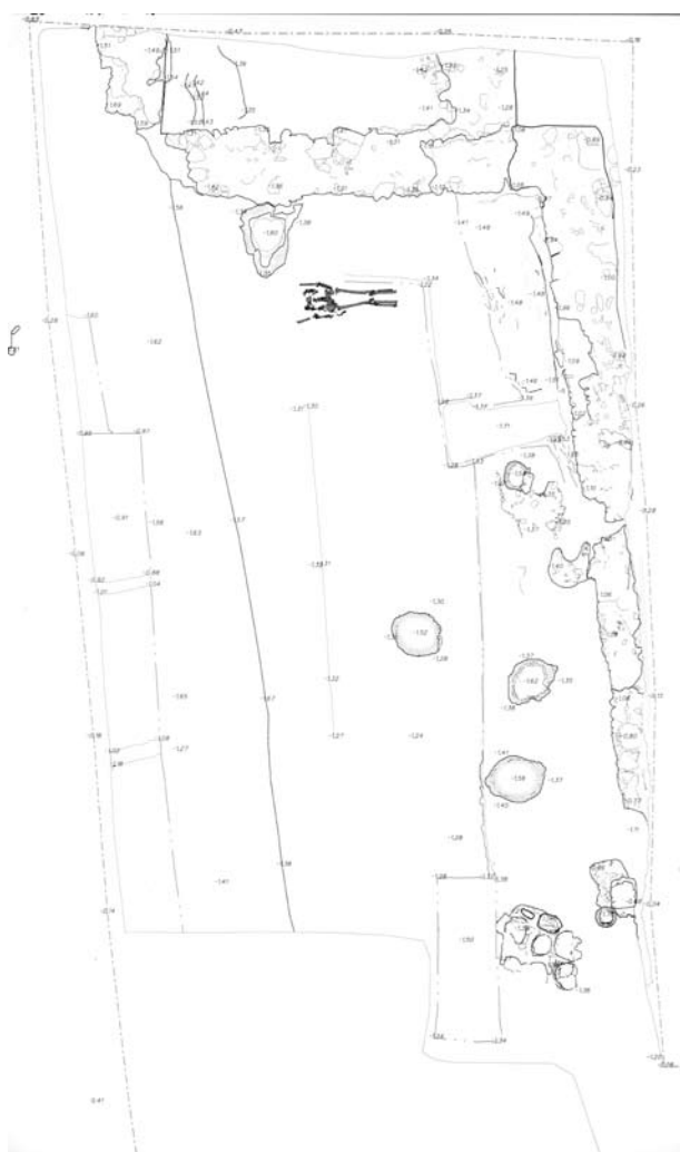
10. A nyugati kolostorszárny alaprajza, az Árpád-kori faépületek cölöplyukaival a 2003/8. szelvényben
