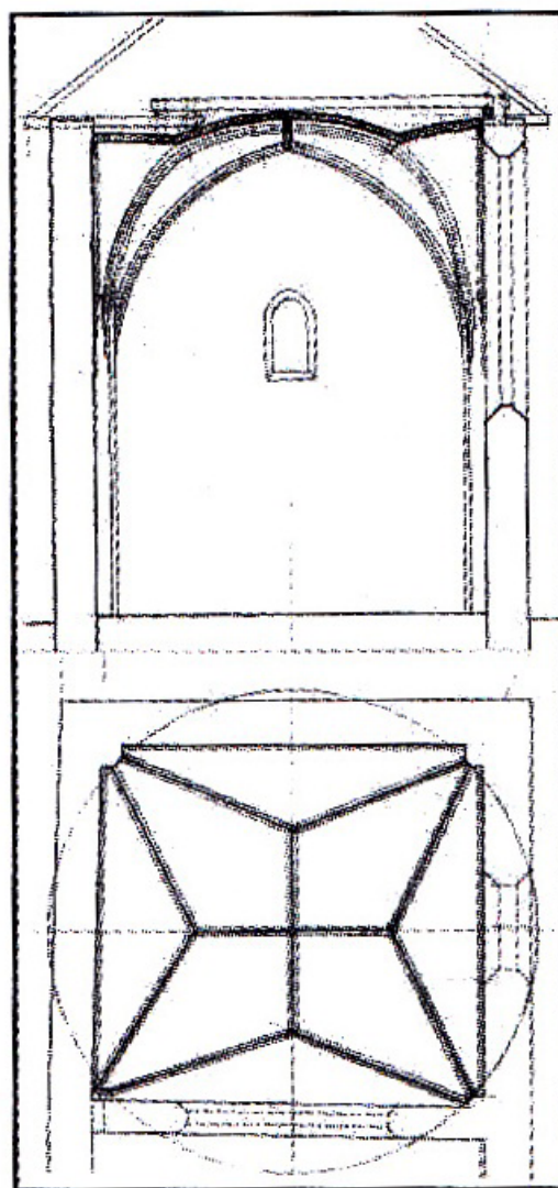
24. Pattantyús Ádám rekonstrukciós rajza (Pálos 2010, 113.)
