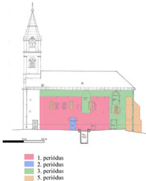
13. Építési periódusok a déli homlokzaton (Forster Tervtár 40535. számon található F-07 jelzetű felmérés felhasználásával)
