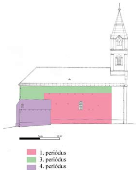
15. Építési periódusok az északi homlokzaton (Forster Tervtár 40535. számon található F-06 jelzetű felmérés felhasználásával)
