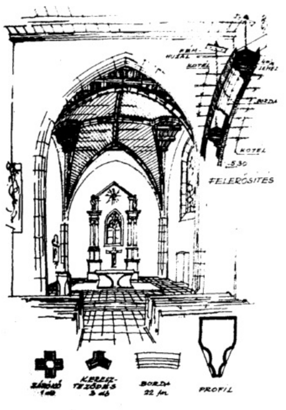
23. Sedlmayr János terve a szentély elpusztult boltozatának helyreállításához, 1976 (Sedlmayr 1979, 170. 17. kép)
