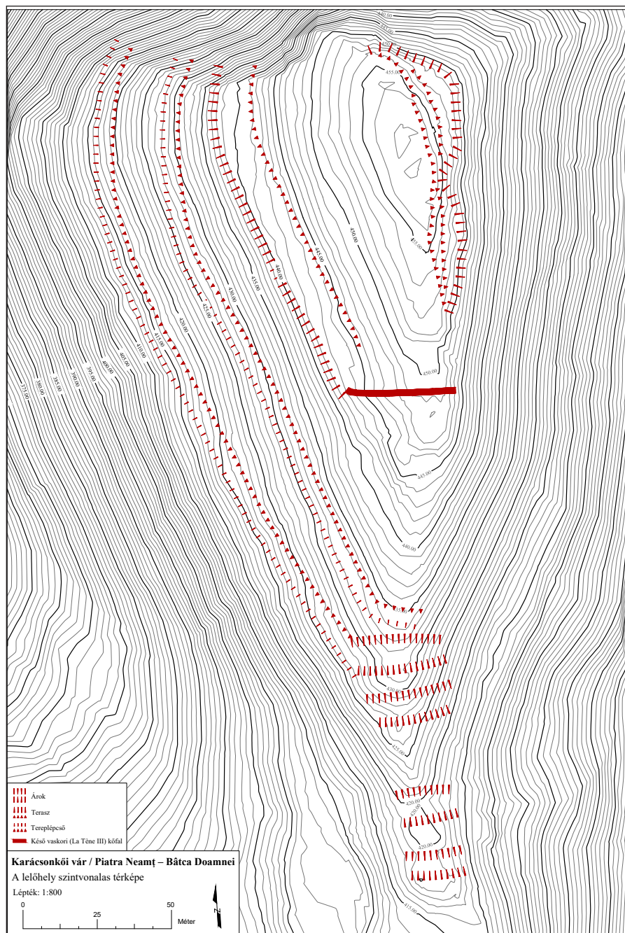
8. kép. A várhegy szintvonalas felmérése (a szerző és a CloudScale Digital Kft. munkája)
