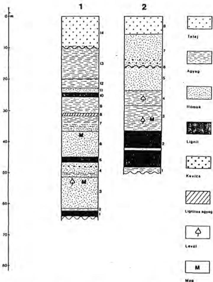
1. ábra: A lelőhelyek földtani szelvénye: 1 = Visonta, NY-i bánya; 2 = Bükkábrány, lignitkölfejtés.
