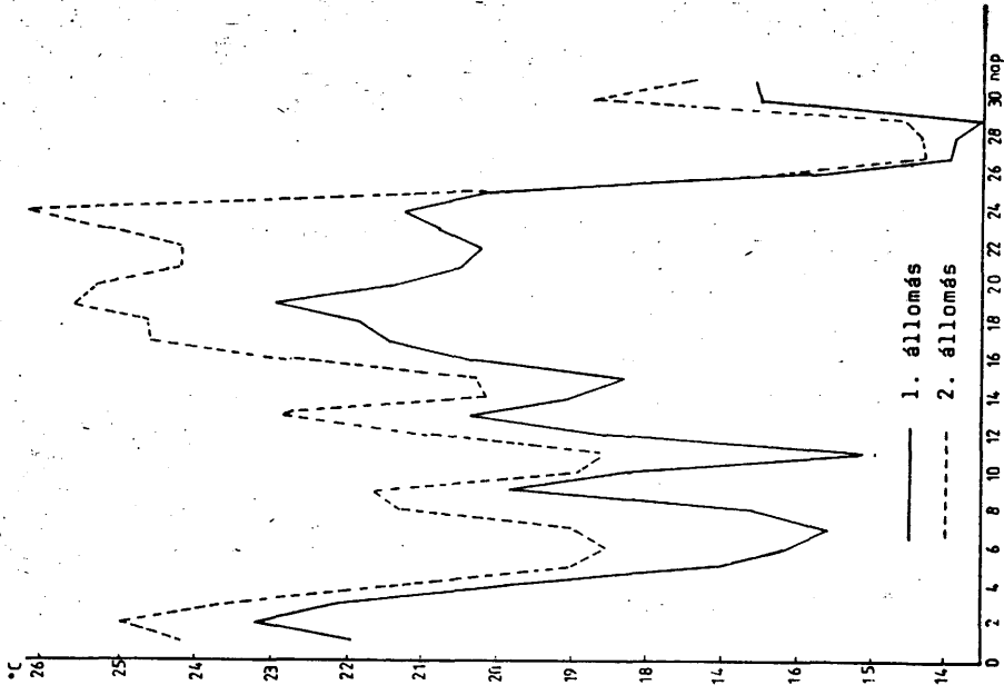
11. ábra. A hőmérséklet havi járása 5 cm magasságban az 1. és a 2. állomáson 1987. júliusában.
