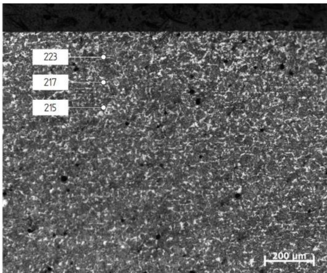
8. ábra: C45 4. minta szövetképe keménységi adatokkal
