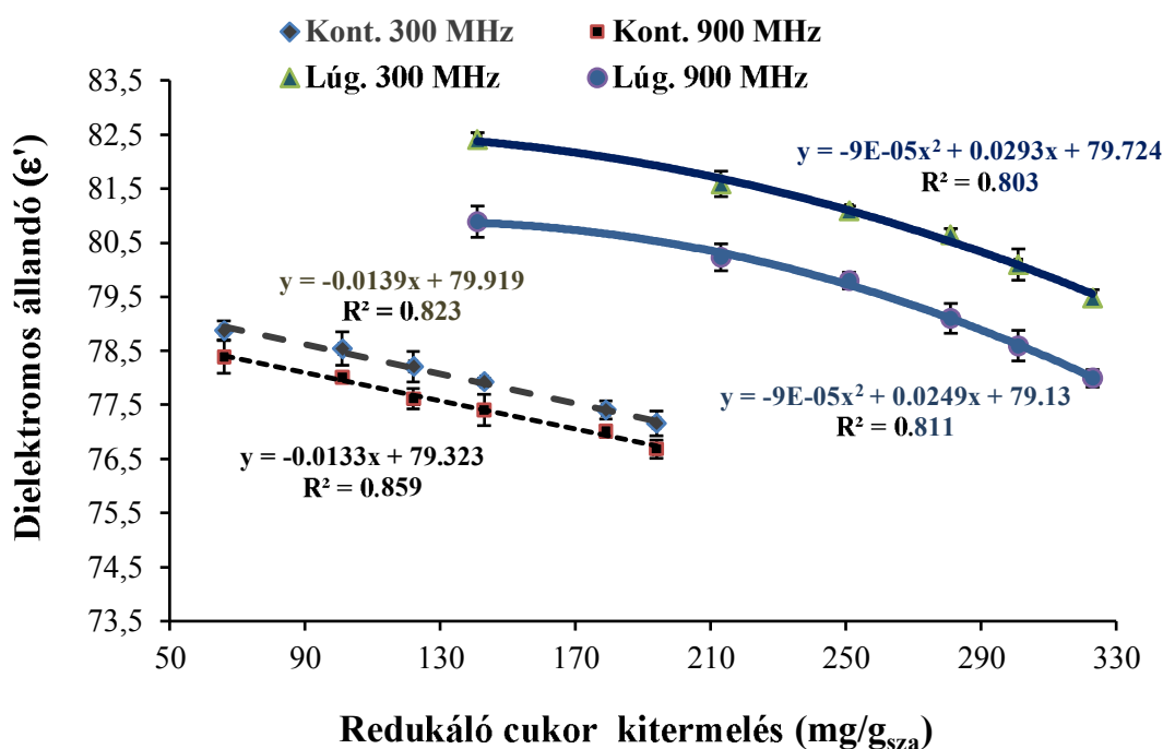
4. ábra – A redukáló cukor kitermelés és a dielektromos állandó (300 MHz ill, 900 MHz) kapcsolata a kezelt és kezeletlen növényi örlemények enzimes emésztése során
