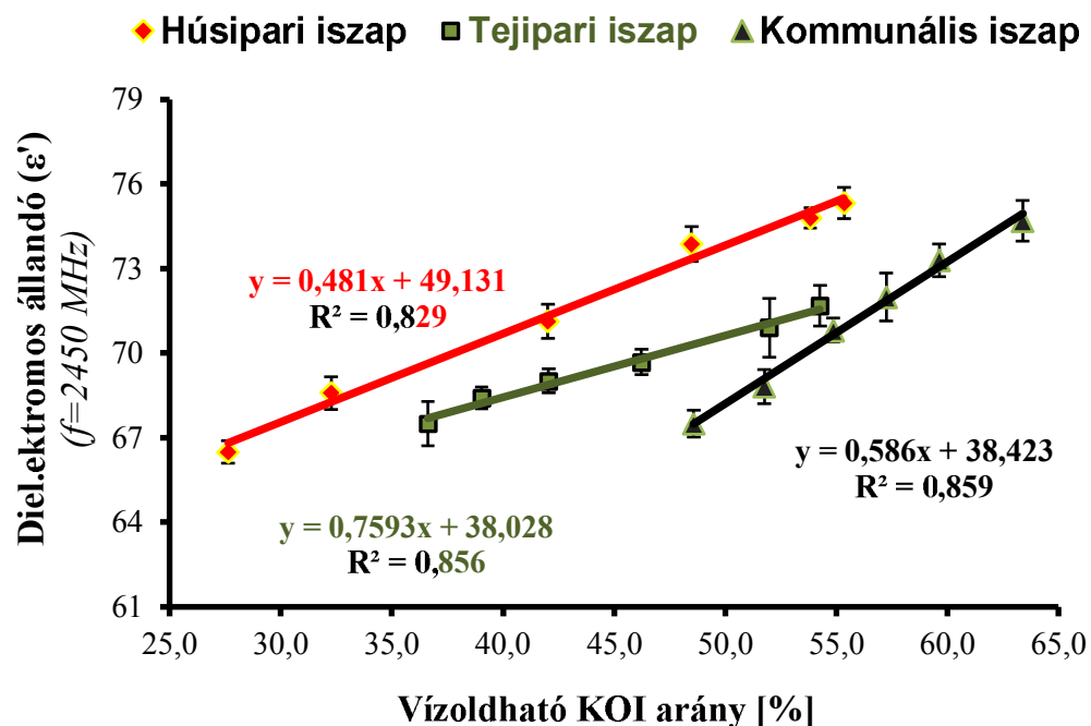
2. ábra – A vizoldható KOI arány és a dielektromos állandó összefüggései a vizsgált szennyvíziszap-típusoknál
