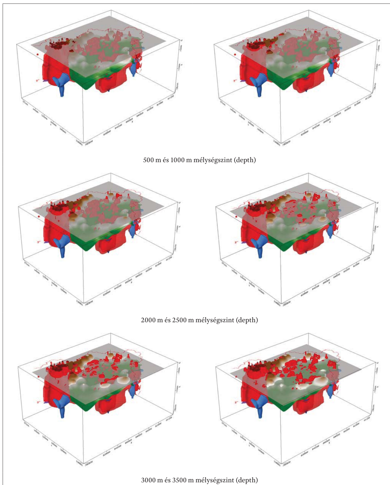
12. ábra A térbeli mágnesezettségi paraméter légi adatokból (piros színnel, \epsilon_r > 0,015 határérték szint), valamint a földi ( \epsilon_r > 0,045 határérték szint) mélységszintekkel (szürke síkfelületek az 500, 1000, 2000, 2500, 3000 és 3500 m mélységben), a szeizmikus prekainozoos medencealjzat szint (zöld-fehér-barna színskála mellett), valamint a kürtő és kaldera csatornák (kék színnel)
