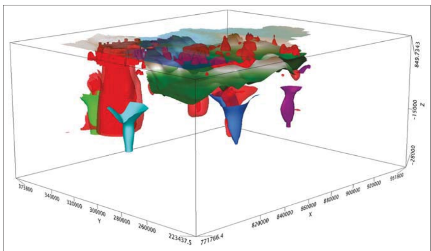
16. ábra Fontosabb vulkánmorfológiához kapcsolható térbeli testek a szeizmikus nagy sebességű medencealjzat szinttel (zöld-barna színnel) és átlátszó felszíni domborzattal. Saványú vulkanitok kürtő–kaldera formák: zöld – Telkibánya–Gönc, világoskék – Szerencs, sötétkék – Nyíregyháza-D, lila – Nagyecsed. Bázisosabb vulkanitok kítőresi központjai (intrúziók, szubvulkánok, vulkánok) piros színnel, az ábrán balról jobbra, Telkibánya, Regéc–Erdőbénye, Kisvárdá és Nyíregyháza-D
