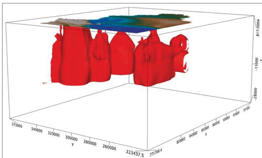
10. ábra | Relatív mágnesezettségi határfelület ( \epsilon_r = 0,045 ) a domborzattal (Regéc, Kisvárdától, Nyíregyháza-D, Nagyecsed központok) Figure 10 | Relative magnetization interface ( \epsilon_r = 0,045 ) with the topography (Regéc, Kisvárdától, Nyíregyháza-D, Nagyecsed centres)
