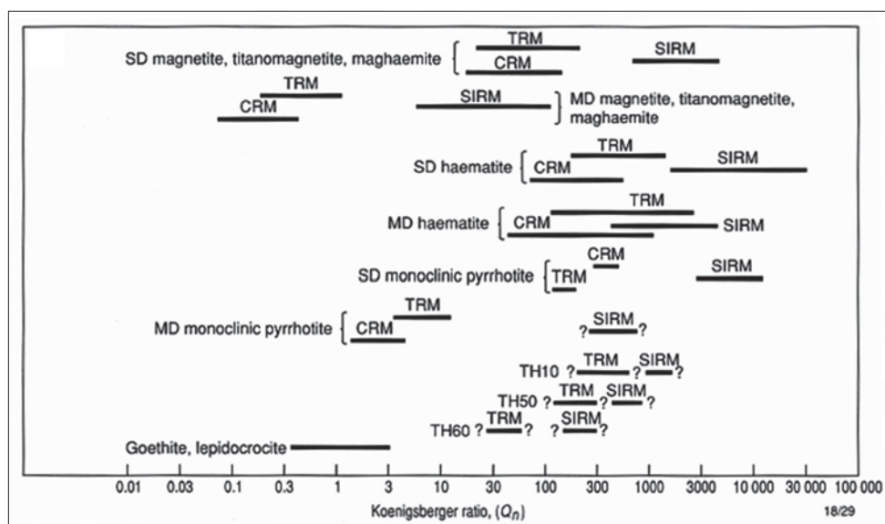
16. ábra Königsberger-arány a főbb mágneses ásványok esetén (Clark 1997) (CRM = kémiai remanens mágnesezettség, TRM = termoremanens mágnesezettség, SIRM = telített izotermikus remanens mágnesezettség, SD = egydomén, MD = multidomén)
