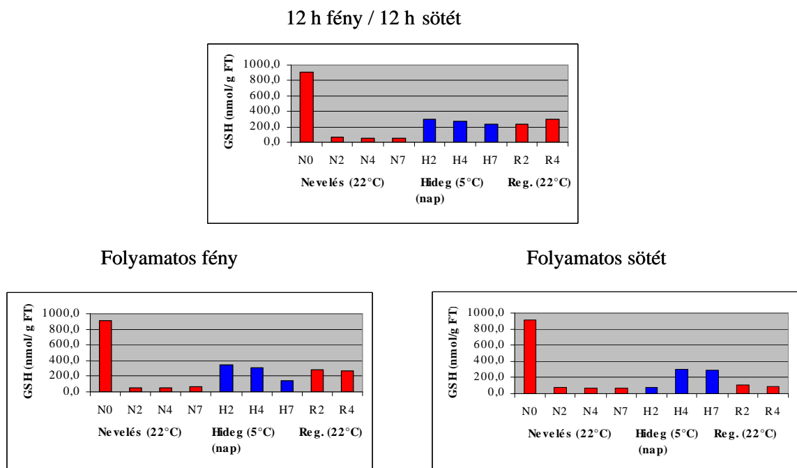
3. ábra. A megvilágítás hidegkezelés és a hatása a redukált glutation (GSH) mennyiségére.
