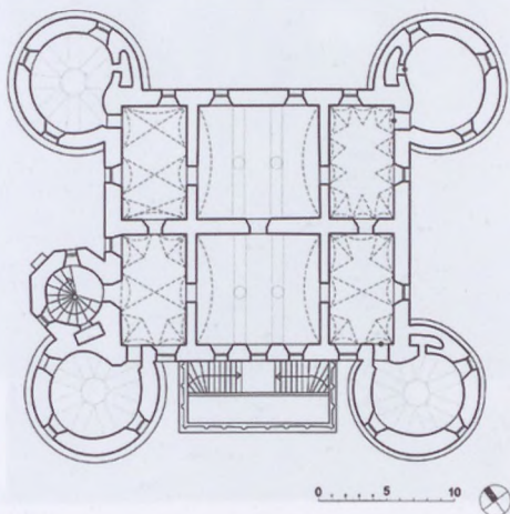
3. II. emeleti alaprajz
