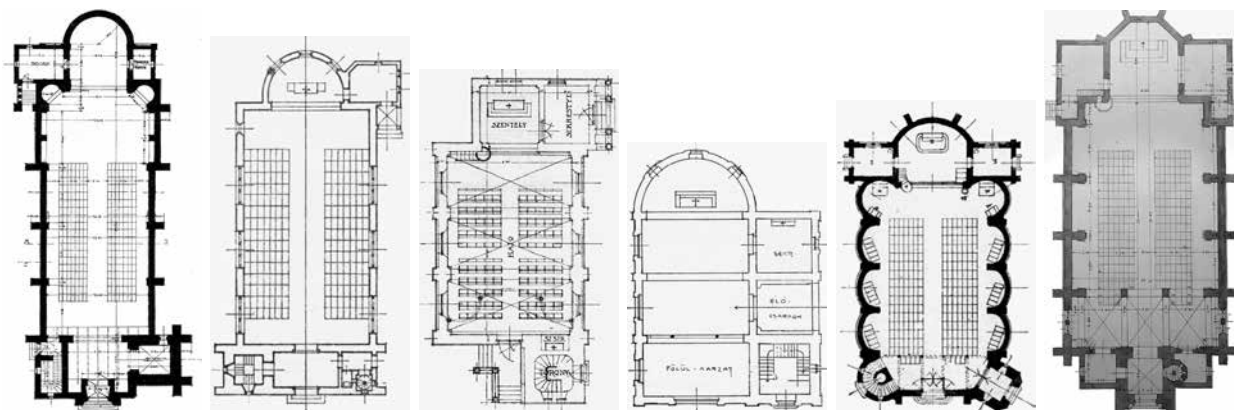
9. Alaprajzi megoldások a pályázatokon – egyhajós: A: Moravec Zsigmond: I.N.D., puszta templomok, Magyar Pályázatok II. 1904/7. 16 – B: Riemer Márkus: Anima,oteles templomok. Magyar Pályázatok II. 1904/3. 9 – C: Goll Elemér: (Kettős kereszt piros mezőben),oteles templomok. Magyar Pályázatok II. 1904/3. 8 – D: Foerk Ernő – Sándy Gyula: Vakolat,oteles templomok. Magyar Pályázatok II. 1904/3. 7 – egyhajós, kápolnasor megidézésével: E: Schneider Iván: Üdvözlégy Mária,oteles templomok. Magyar Pályázatok II. 1904/3. 25 – F: Szilágyi János: Genitore-genitoque, puszta templomok. KFL VIII.3.a. 9.
