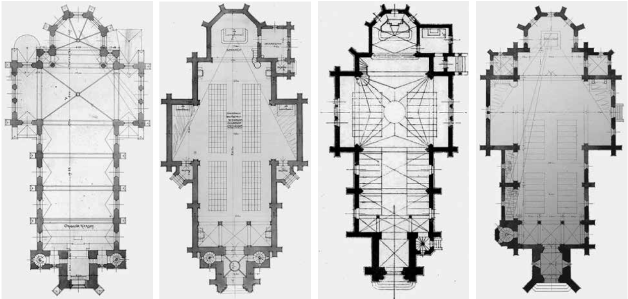
7. Alaprajzi megoldások a pályázatokon – egyhajós latinkereszt: A: Károlyi Emil: K. E., pusztai templomok. KFL VIII.3.a. 11/h. – B: Bánszky Mihály – Sautner Félix: Üdvözlégy Mária, pusztai templomok. KFL VIII.3.a. 12. – C: Schuldner Miklós – Wannemacher Fábrián: In nomine Patris, pusztai templomok, Magyar Pályázatok II. 1904/7. 15 – D: Ybl Lajos: Glória, pusztai templomok. KFL VIII.3.a. 14.
