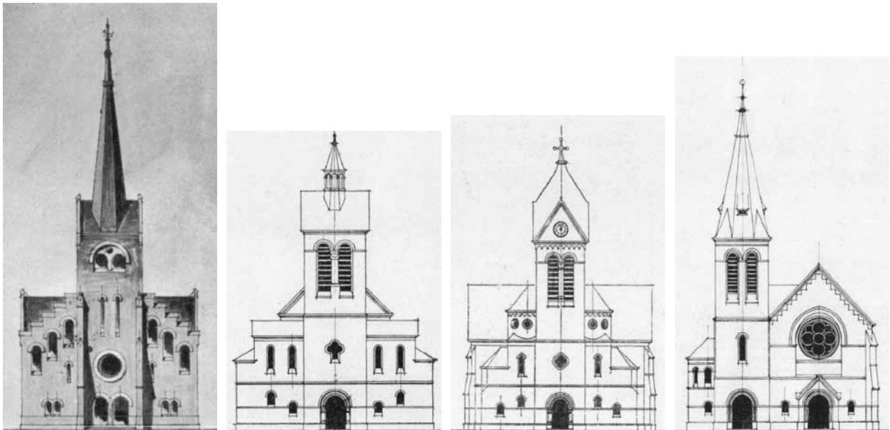
4. Homlokzati- és tömegmegoldások változatai a tárgyalt pályázatokon: középtornyos egyszerűsített és aszimmetrikus tornyos, egyszerűsített: A: Riemer Márkus: Exelsior, telepes templomok. Magyar Pályázatok II. 1904/3. 17 – B: Miklós Ede: Evangelium B, telepes templomok. Magyar Pályázatok II. 1904/3. 18 – C: Miklós Ede: Reformáció, telepes templomok. Magyar Pályázatok II. 1904/3. 21 – D: Miklós Ede: Luther A, telepes templomok. Magyar Pályázatok II. 1904/3. 10
