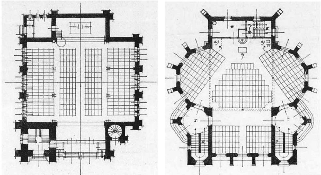
12. Centrális megoldások református templomokra: A: Károlyi Emil: (Vörös pont kék körben), telespes templomok. Magyar Pályázatok II. 1904/3. – B: Schneider Iván: Miatyánk, telespes templomok. Magyar Pályázatok II. 1904/3. 12
