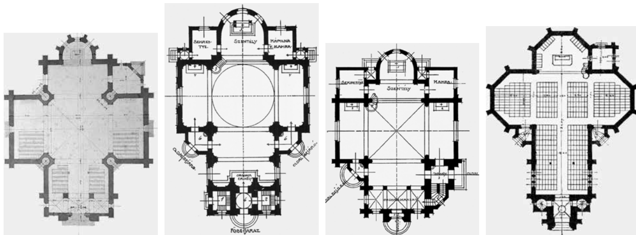
8. Alaprajzi megoldások a pályázatokon – centralizáló.: A: ifj. Bobula János: (Szent György legyőzi a sárkányt), puszta templomok. KFL VIII.3.a. 13. – B: Opaterny Flóris – Bohn Alajos: Oremus (első variáns), puszta templomok, Magyar Pályázatok II. 1904/7. 14 – C: Opaterny Flóris – Bohn Alajos: Oremus (második variáns), puszta templomok, Magyar Pályázatok II. 1904/7. 15 – D: Bánszky Mihály: Luther, telepes templomok. Magyar Pályázatok II. 1904/3. 6
