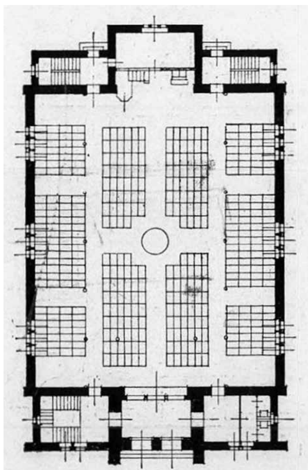
13. Centrális megoldások református templomokra: A: Riemer Márkus: Exelsior , telepes templomok. Magyar Pályázatok II. 1904/3. 17 – B: Walch Viktor – Borsos József: Szeretet . Magyar Pályázatok II. 1904/3. 19
