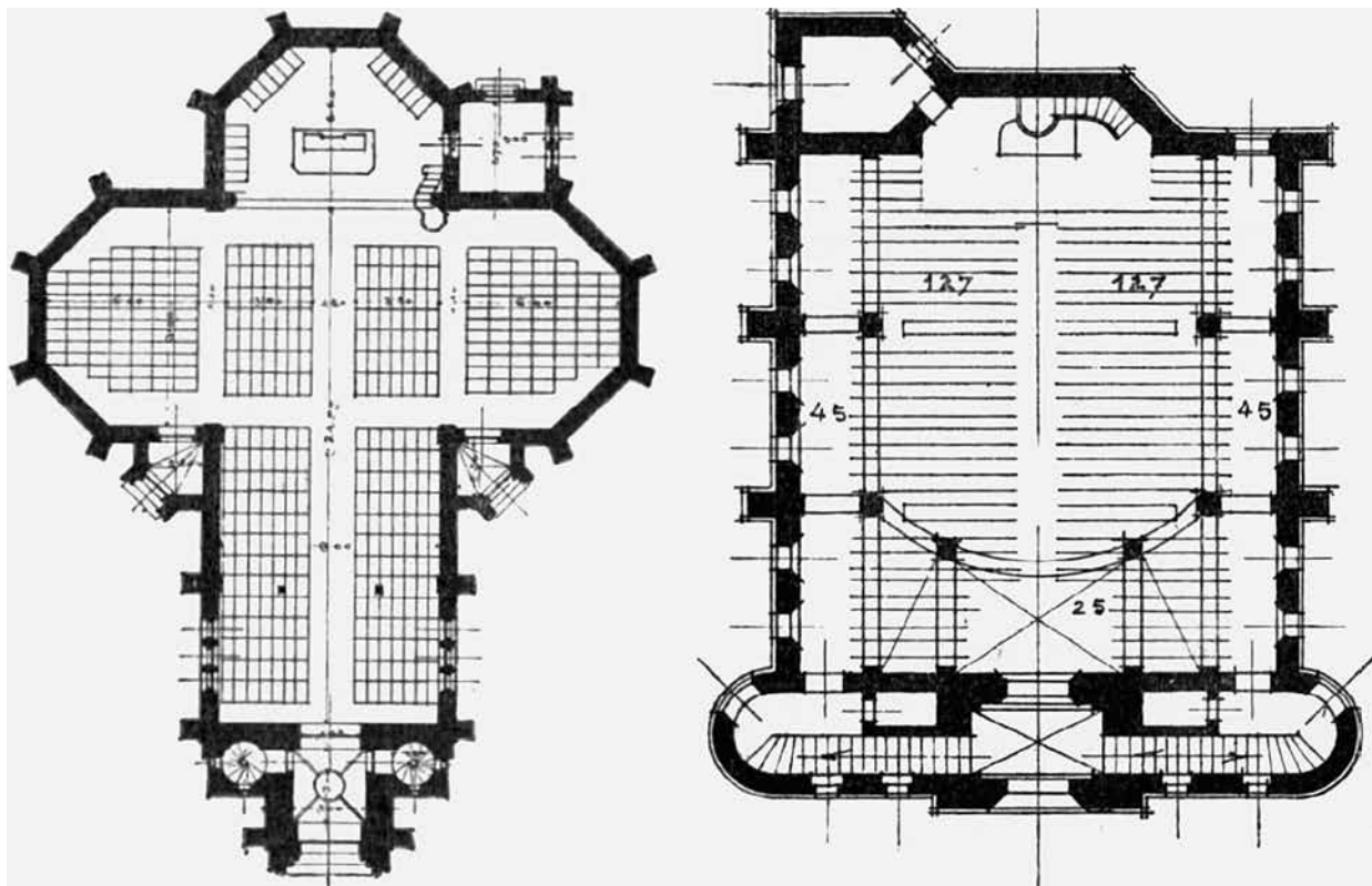
11. Evangélikus és református templom jellegzetes alaprajza: A: Bánszky Mihály: Luther, telepes templomok. Magyar Pályázatok II. 1904/3. 6 – B: Miklós Ede: Reformáció, telepes templomok. Magyar Pályázatok II. 1904/3. 21
