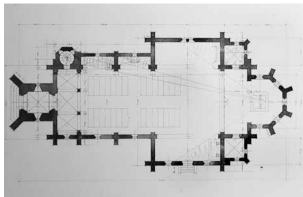
14. A szabadkai pályázatra Ybl Lajos által készített: Glória és Károlyi Emil: KE jellegű tervének alaprajza, rajtuk dr. Révai Tibor jelöléseivel; a látószög vonalaival és az általa szükségtelennnek, rossznak tartott térrészek besatírozásával: A: Károlyi Emil: KE, pusztai templomok. KFL VIII.3.a. 11/h – B: Ybl Lajos: Glória, pusztai templomok. KFL VIII.3.a.14.
