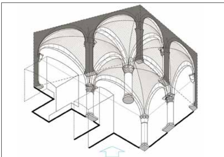
5. kép A Szent István-terem izometrikus képe (Borosházi Tamás szerkesztése, Vukov 2004, 90. kép)
