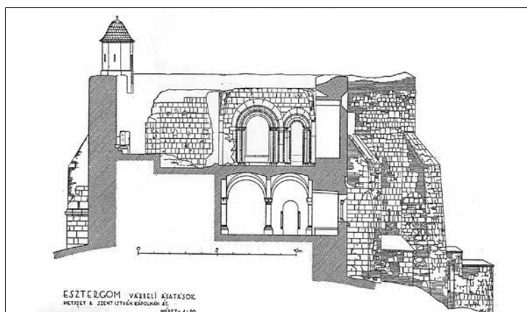
4. kép A királyi palota kelet-nyugati metszete a Szent István-teremen és a kettős kapus termen át (Lux Géza alapján)
