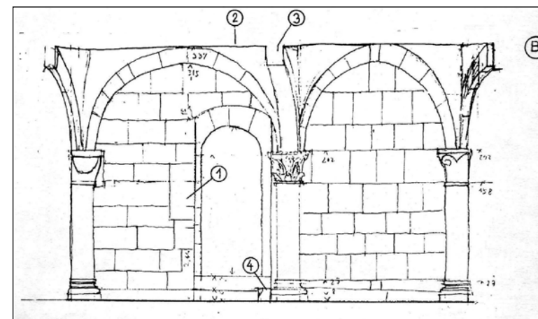
9. kép A Szent István-terem kelet felé, metszetrájk (Vukov Konstantin felmérése, 1990)
