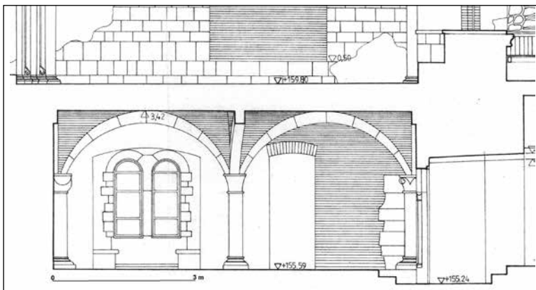
6. kép A Szent István terem nyugat felé, metszetrájk (Vukov Konstantin felmérése, 1990)
