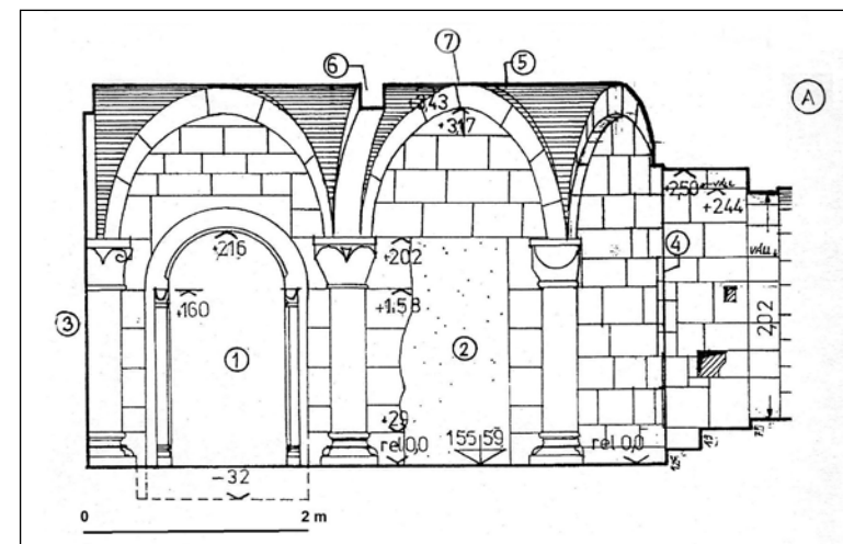
8. kép A Szent István- terem észak felé, metszetrájk (Vukov Konstantin felmérése, 1990)
