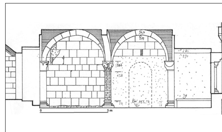
7. kép A Szent István-terem dél felé, metszetrájk (Vukov Konstantin felmérése, 1990)
