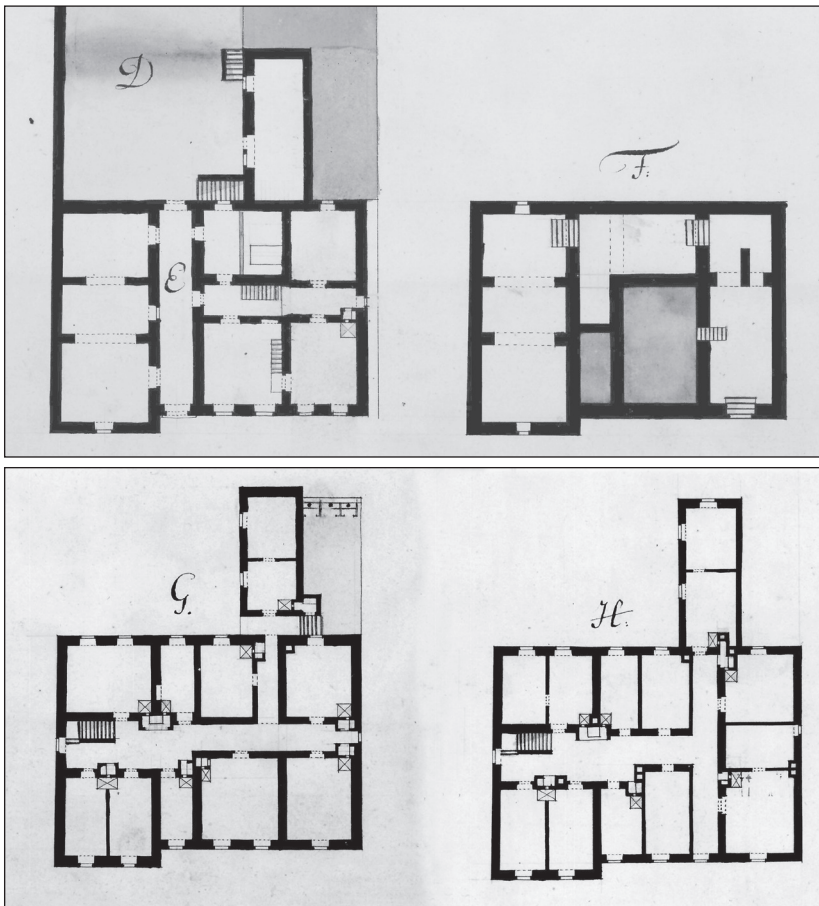
1/a ábra: A Kolleum alaprajza (1773 után, részletek)
