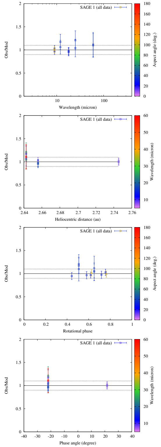
Fig. B.13. (308) Polyxo.
