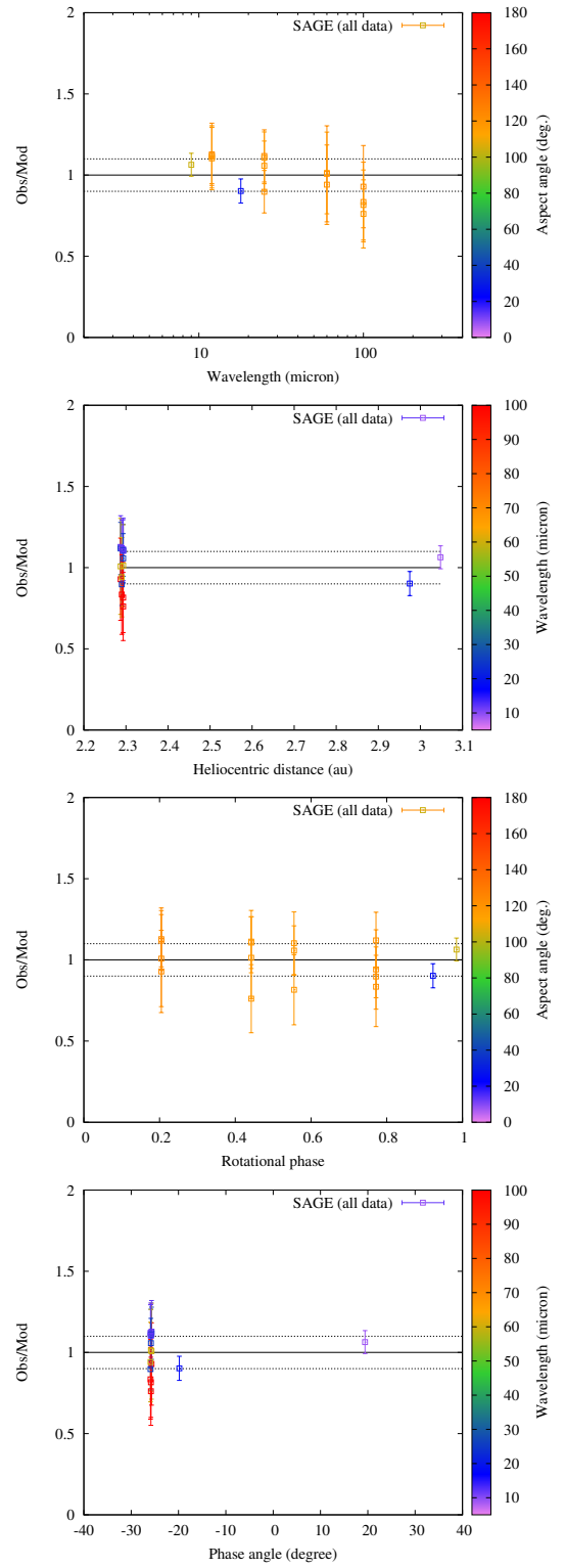
Fig. B.11. (145) Adeona.
