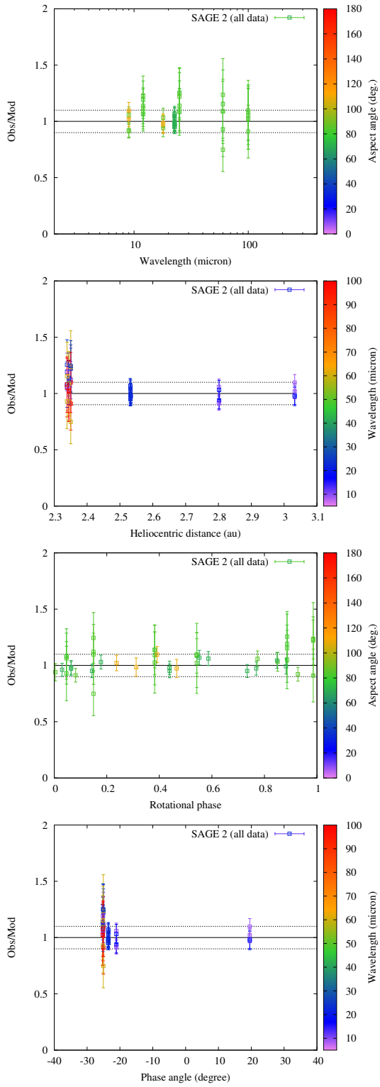
Fig. B.10. (114) Kassandra.
