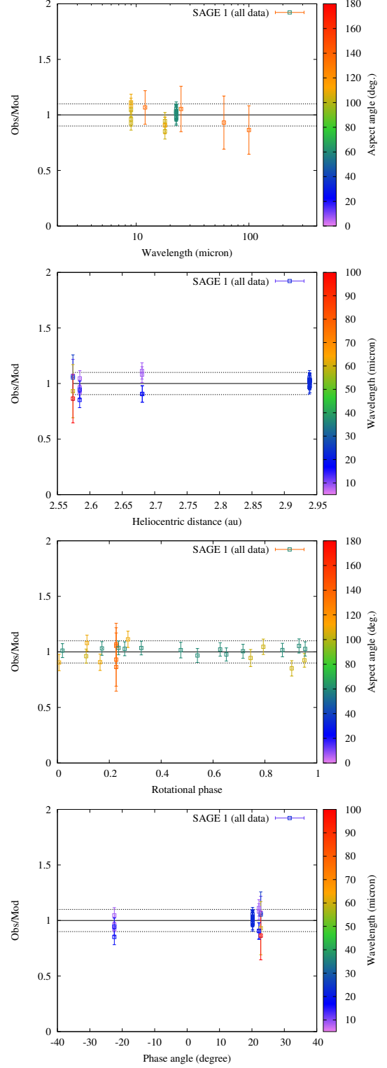
Fig. B.15. (441) Bathilde.
