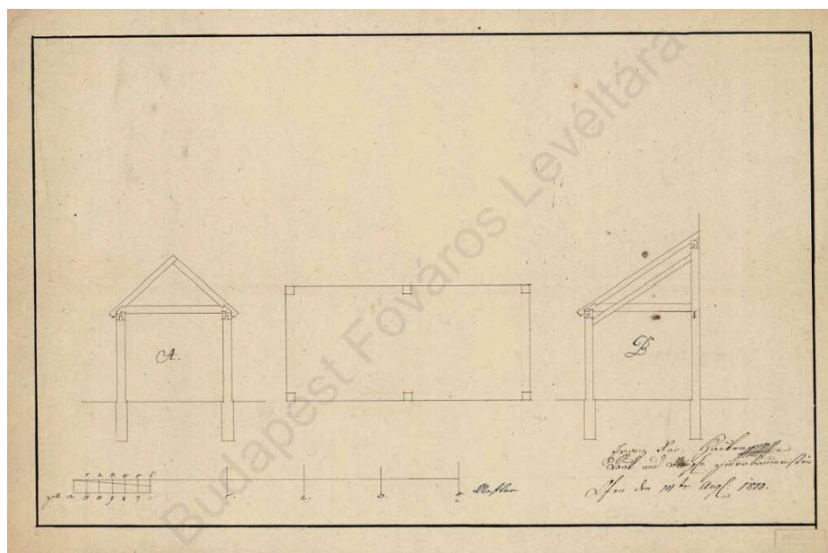
4. kép. Franz Xaver Hacker ácsmester terve tűzoltókocsi tárolására alkalmas kocsiszínre, 1800. (BFL XV.17.a.302 Nr. 103.)
