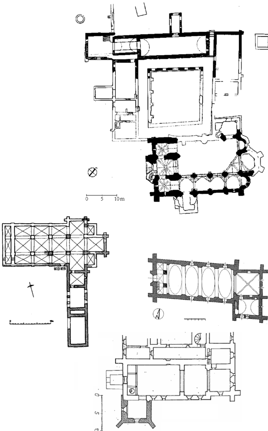
2. ábra. Premontrei prépostságok megkutatótt alaprajzai II.: Zsámbék, Gyulafirátót, Mórchida, Túróc
