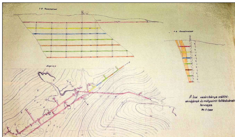
A licei bánya szállítóaknájának és további feltárásának a tervrajza. 111 (Fotó: Breznanik Peter.)
