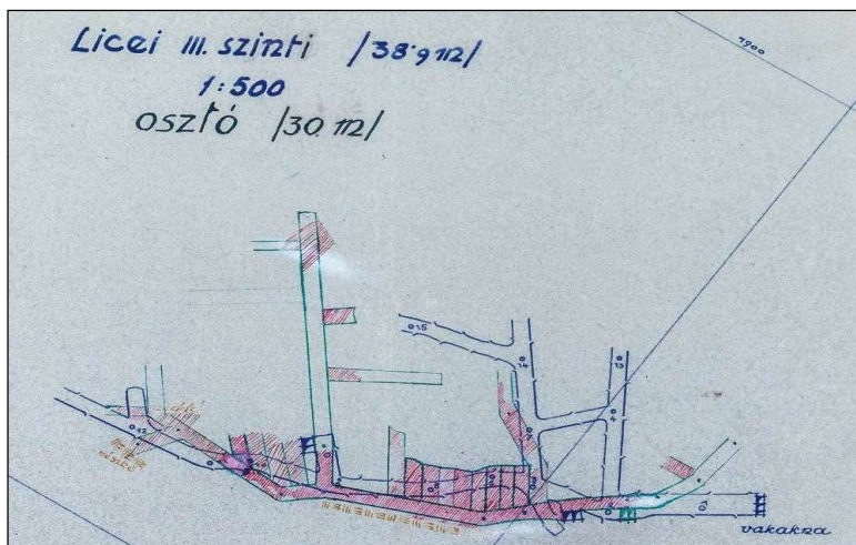
A 30-as osztószint térképe. 110 (Fotó: Breznanik Peter.)
