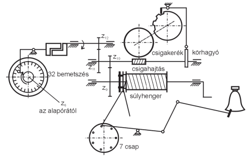
13. ábra. Az ütésekkel jelző modul kinematikai rajza
