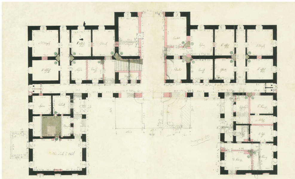
A székház földszinti alaprajza MNL JNSZML Tervtár V. 84.
