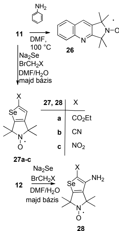
5. Ábra. Kinolinnal és szelenofénnel kondenzált pirrolin-nitroxid szintézise.
