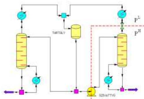
4. ábra Dupla oszlopos szakaszos sztripper
