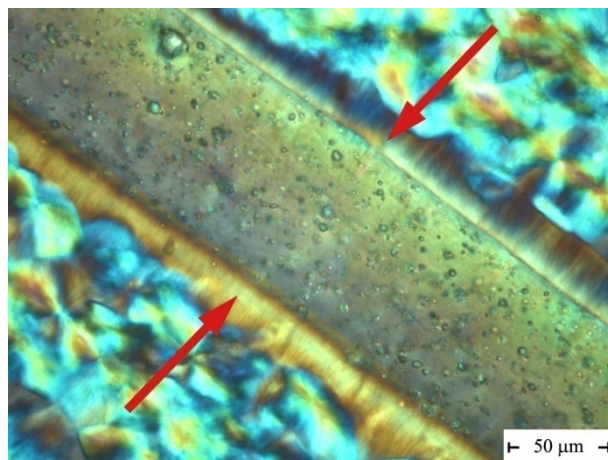
7. ábra A szál/mátrix határfelületén kialakuló transzkristályos réteg beta-PP alapú kompozit esetében 172°C-on préselve
