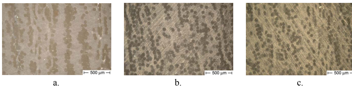
3. ábra Keresztmetszeti csiszolatok fénymikroszkópos felvételei, 170°C-on konzolidált lapok esetében: (a) \beta -PP – 0,3 g/10 perc, (b) rPP – 12 g/10 perc, (c) rPP – 45 g/10 perc
