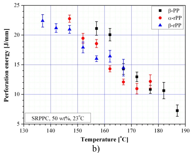
8. ábra Szakító szilárdság (a), illetve a perforációs energia a préselési hőmérséklet függvényében
