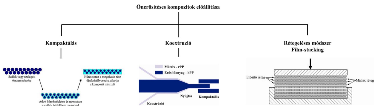
1. ábra Különböző önerősítéses kompozit gyártási technológiák
