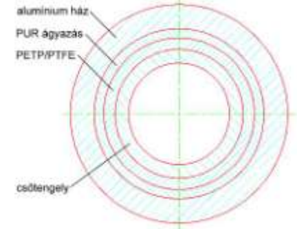
Javasolt re-konstrukció hibrid ágyazással
