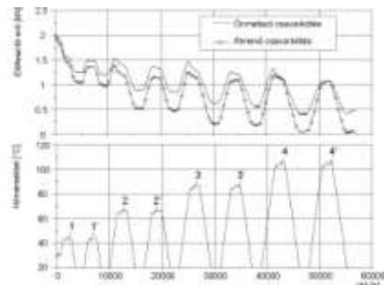
Az előfeszítő erő változása ciklikus hőterhelés esetén
