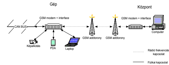
A kétirányú adatátviteli rendszer vázlata
