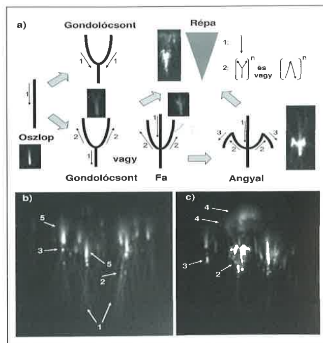
3. ábra. (a) Vörös lidérek jellemző alakjai és az ezeket kialakító kisülési frontok terjedésének irányai. A számok a kisülési frontok megjelenésének egymásutánosságára utalnak. (b)-(c) Vörös lidérek különböző gyakorisággal megfigyelhető alakjait: 1. indák (tendrils), 2. gyöngyök (beads) a lidérc indái mentén vagy a fényes testben, 3. foltok (spots) közvetlenül a fényes lidérc test alatt, 4. puffok (puffs), 5. parázlás (glow) a fényes test körül
