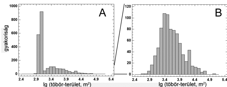
6. ábra: Töbörterületek eloszlásfüggvénye a szimbólumszerű töbrökkel együtt az összes (A) és azok nélkül (B) Fig. 6: Distribution function of doline area: all with symbolic dolines (A) and without them (B)
