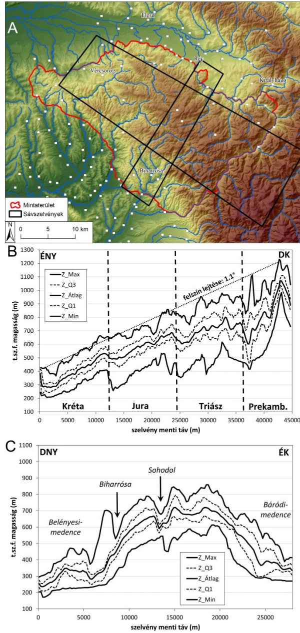
3. ábra: Sávsvélvények a Királyerdőn keresztül. A: sávsvélvények helye; B: ÉNy-DK-i sávsvélvény (alul a domináns kőzet időszak); C: ÉK-DNy-i sávsvélvény
