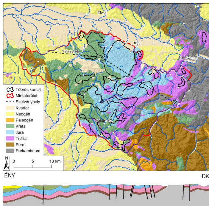
1. ábra: A Királyerdő geológiai térképe és ÉNY-DK-i geológiai szelvénye (GIUȘCĂ – BLEAHU, 1967 felhasználásával)
