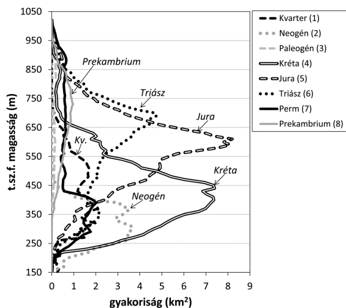
4. ábra: Az egyes földtörténeti korokban képződött kőzetek mai t.sz.f. magassága
