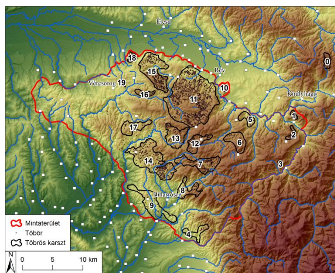
8. ábra: A töbrös felszínek elhelyezkedése a Királyerdőben
