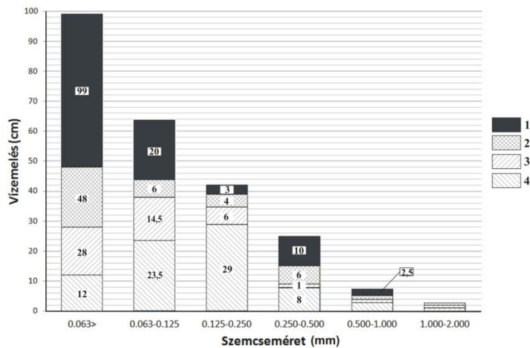
2. ábra: A vízelőképeség az idő- és a szemcseméret függvényében Jelmagyarázat: 1. teljes vízelőelés, 2. 24 órás vízelőelés, 3. 5 órás vízelőelés, 4. 1 órás vízelőelés Fig. 2: Water lifting ability in the function of time and grain size Legend: 1. total water lifting, 2. 24-hour water lifting, 3. 5-hour water lifting, 4. one-hour water lifting
