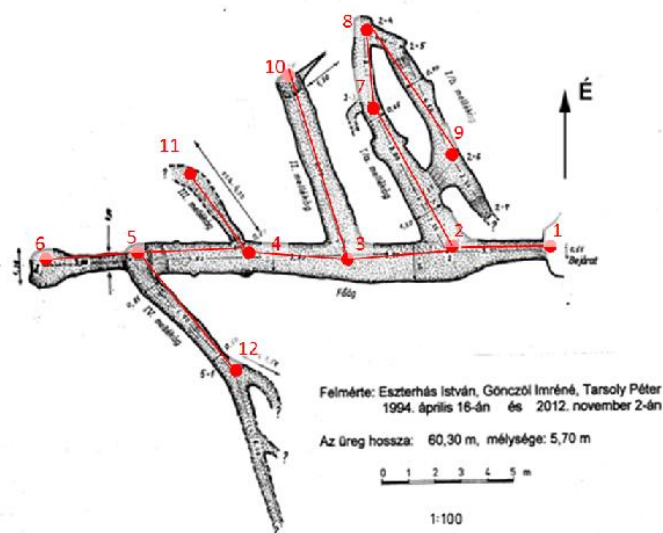
8. ábra A Bárcaházi-barlang drótmodellje Fig.8. The wire-model of the Bárcaházi-cave
