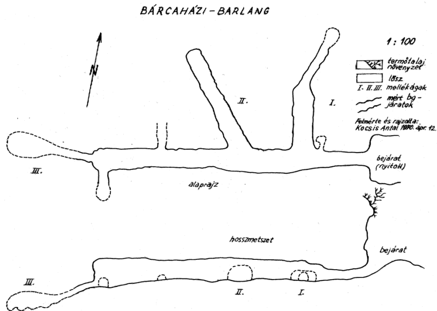
3. ábra Kocsis Antal 1970-ben rajzolt térképe Fig.3. The map of the Bárcaházi-cave, made by Antal Kocsis in 1970
