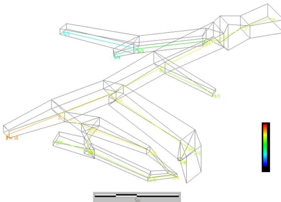
6. ábra A barlang térmodellje a Polygon v. 2 szoftverrel készítve Fig.6. The 3D-model of the Bárcaházi-cave, made by the Polygon v. 2 software
