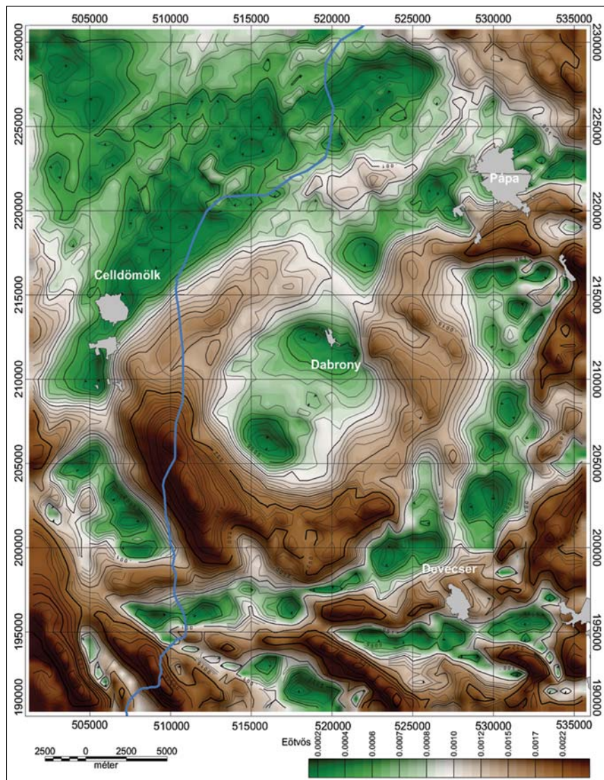
6. ábra | A dabronyi gravitációs anomália horizontálisgradiens-képe a regionális hatások eltávolítása után Figure 6 | Bouguer residual anomaly horizontal gradient map of the Dabronyi gravity anomaly area
