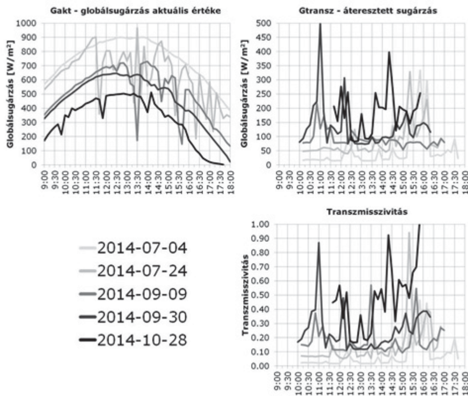
4. ábra A globálsugárzás napi menete az Aesculus Hippocastanum mérési napjain, valamint a faj napsugárzás áteresztőképességének évszakos változása
