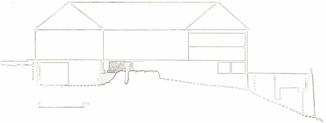
11. kép. K–Ny-i irányú metszet a későközépkori városfaltól a Tánicsics Mihály utcáig Abb. 11. O–W gerichteter Schnitt von der spätmittelalterlichen Stadtmauer bis zur Tánicsics Mihály-Gasse
