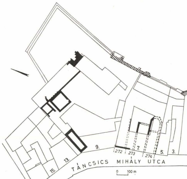
13. kép. A Tánacsics utca 7. és 9. számú telkek és környékük modern helyszínrajza az elvégzett régészeti kutatásoknál feltárt középkori épületmaradványokkal Abb. 13. Moderner Situationsplan der Grundstücke unter Tánacsics Mihály-Gasse Nr. 7 und 9 und ihrer Umgebung mit den anlässlich der archäologischen Forschungen erschlossenen mittelalterlichen Gebäuderesten
