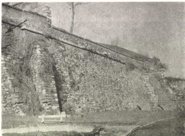
4. kép. Későközépkori várossfal és támpillérei a Tánicsics utca 7. és az Erdélyi bástya között Abb. 4. Spätmittelalterliche Stadtmauer und ihre Stützpfiler zwischen der Tánicsics Mihály-Gasse Nr. 7 und der Erdélyi (Transsilvanischen) Bastei
