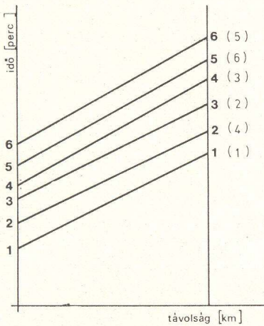
4b ábra. A figyelembevett út-idő diagram
