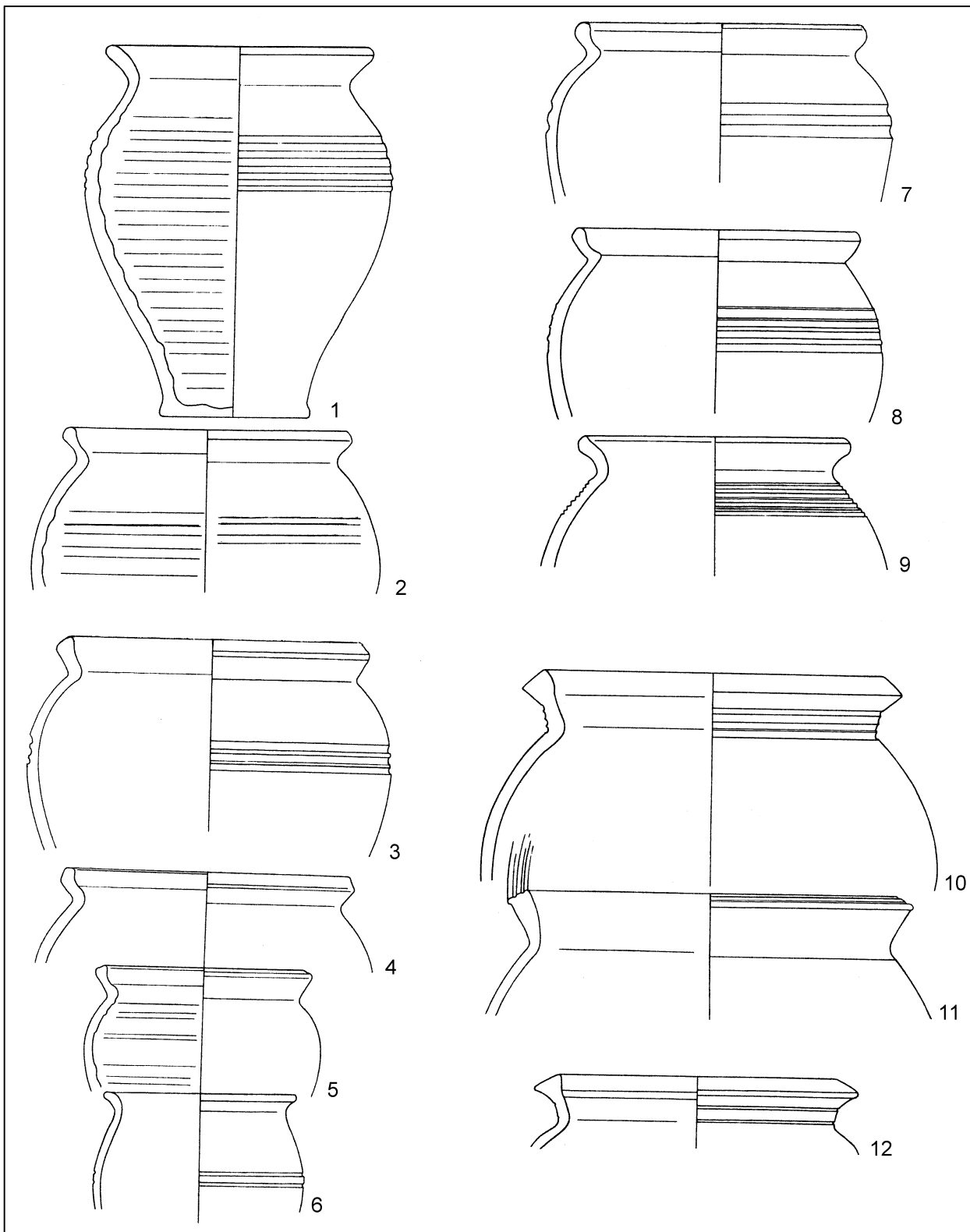
12. kép. Házi kerámiák a kemencék betöltéséből - Fazekak Abb. 12. Hauskeramik aus der Aufschüttung der Öfen - Töpfe M = 1 : 3
