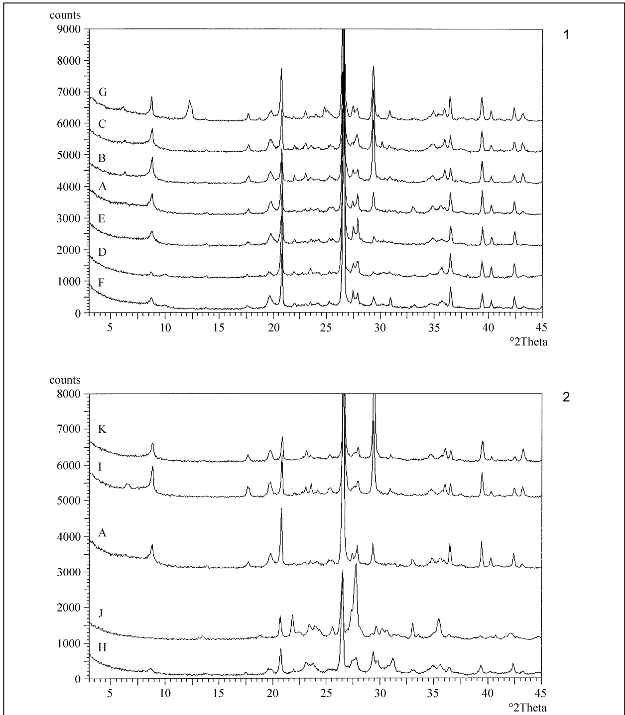
48. kép. Röntgen-diffraktogramok
