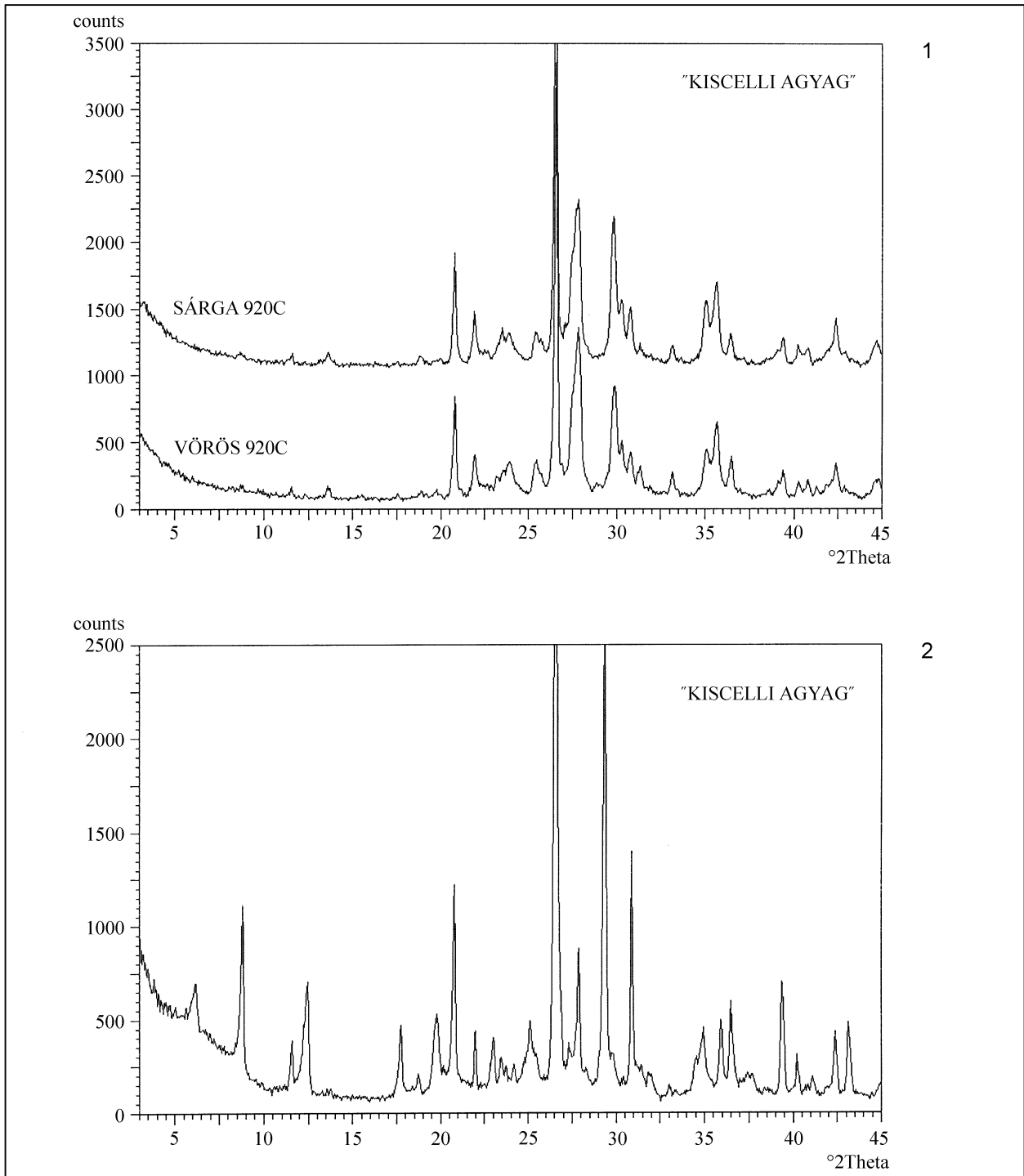
49. kép. Röntgen-diffraktogramok 1. 920 °C-on kiégetett kiscelli agyagminta; 2. Nyers kiscelli agyagminta
