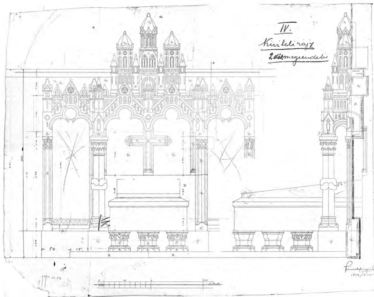
19. A sírépítmény kivitelezési terve. Schulek Frigyes, 1898 (BTM KM ÉGy. ltsz.: 52.41.2863)
