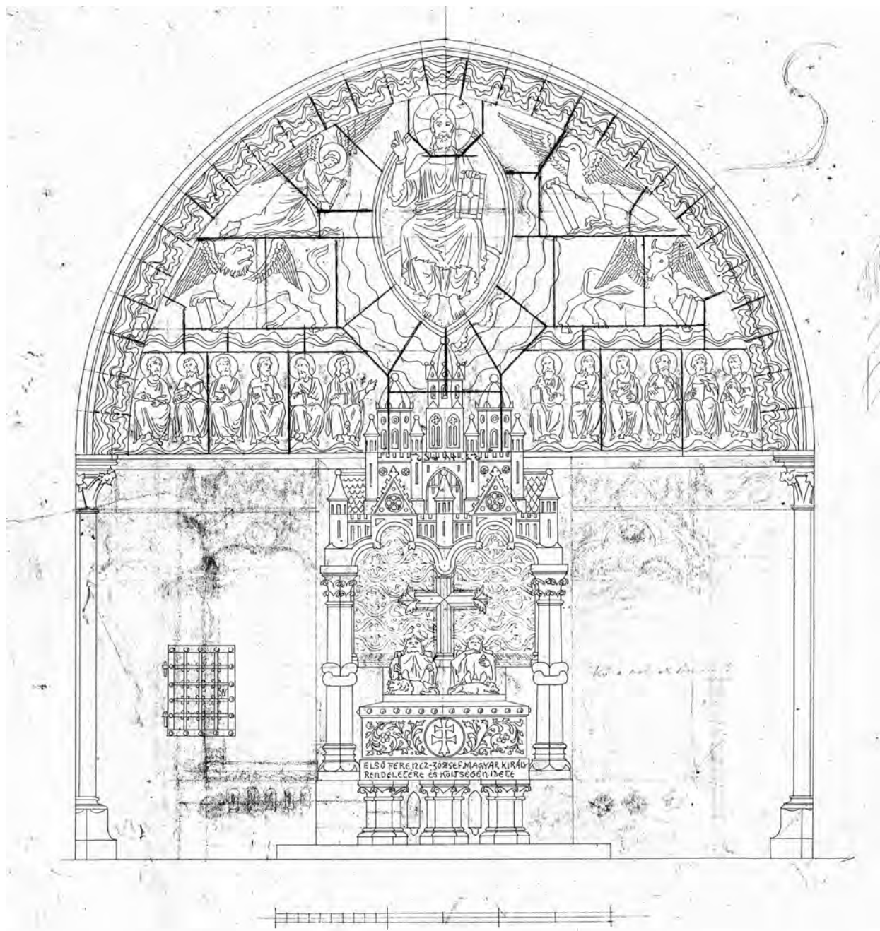
18. A síremlék terve a timpanon kőkiosztásának jelölésével. Schulek Frigyes, 1898 (BTM KM ÉGy. ltsz.: 52.41.625)
