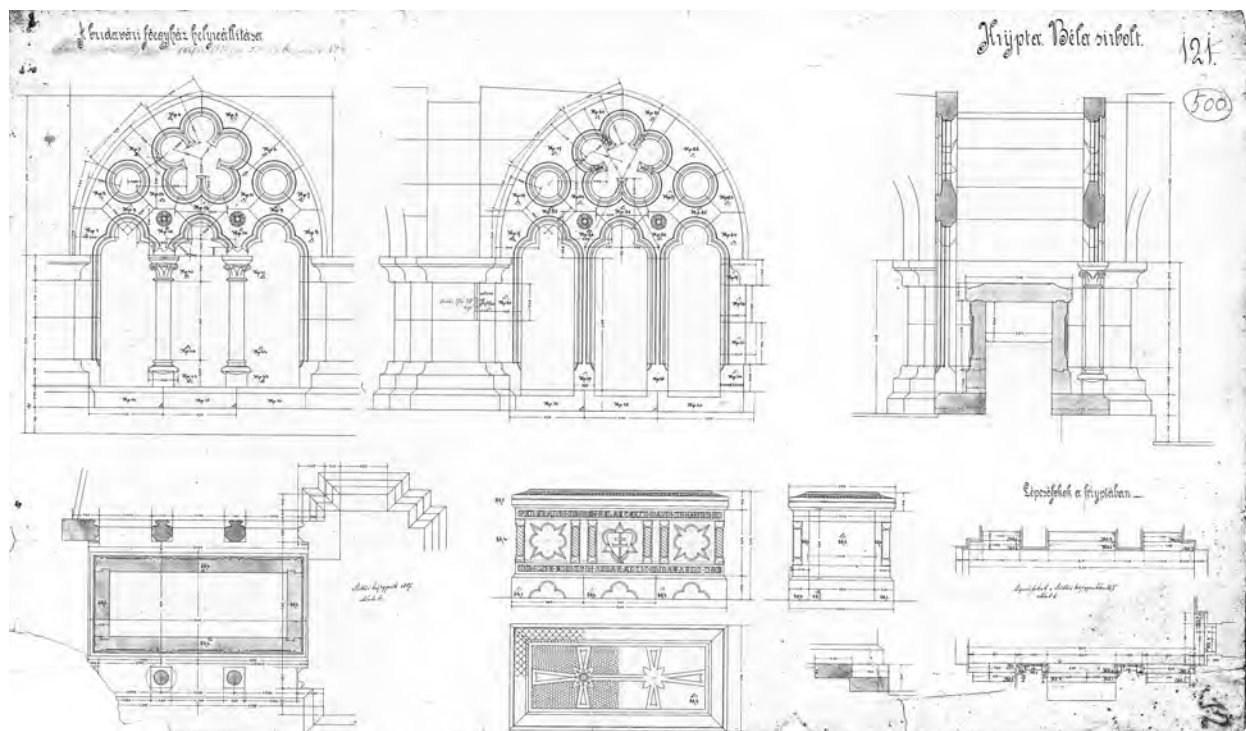
3. Az attemplomban megvalósult síremlék terve, feltehetően Wagner Ferencétől, 1887 (BTM KM ÉGy, ltsz.: 63.21.476)
