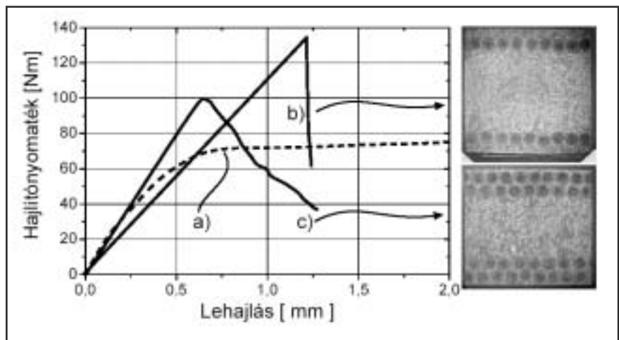
5. ábra. 12 mm vastag lapokból kivett próbatetek hajlítódigramja: (a) erősítés nélküli lapnál, (b) kompozithuzalval 2×1 rétegben erősített, (c) kompozithuzalval 2×2 rétegben erősített szendvicslapoknál
