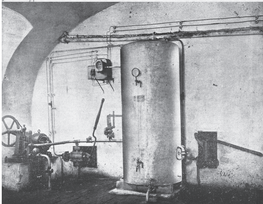
A főgimnázium vízmű berendezése és folyamatábrája az 1913/14-es tanévi értesítőtől
