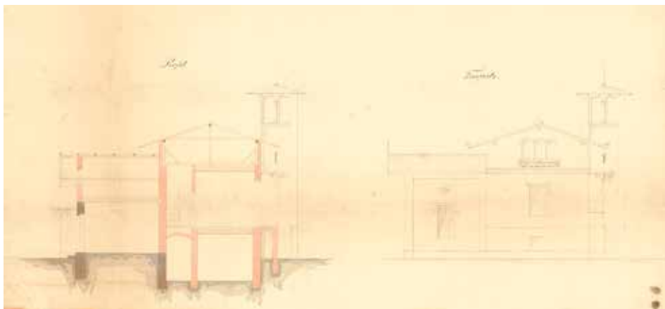
9. kép. A Vankó-villa hosszmetSZete és oldalhomlokzata. Pollack Ágoston, 1846. Forrás: BFL XV.17.b.311 SzB 11522
