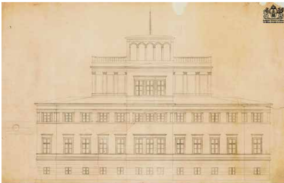
5. kép. Az ikerházi Batthyány-kastély hátsó homlokzatának terve. Pollack Ágoston, Ybl Miklós. 1845. Forrás: BFL XV.17.f.331.b 92/1
