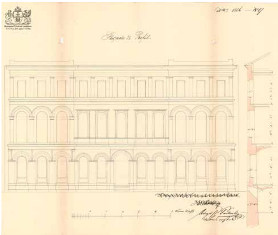
8. kép. Vendelin Péter háza. Pollack Ágoston, 1846. Forrás: BFL XV.17.b.311 SzB 11976-e
