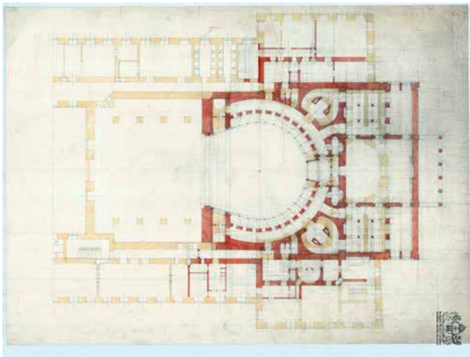
2. kép. A Német színház átépítésének terve. Ybl Miklós, 1840–41 körül. Forrás: BFL XV.17.f.331.b 141/1
