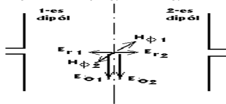
5. ábra. Az antenna-rendszer jósági tényezőjének számításához
