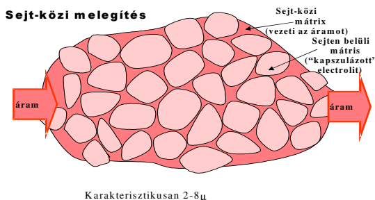
10.ábra. A sejtmembrán elektromos mezőt árnyékoló hatása
