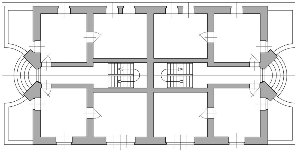
2. kép. Négyosztatú, nyolclakásos ház földszinti alaprajza. (Eredeti tervrajz: MNL NML 18667/1937.)
